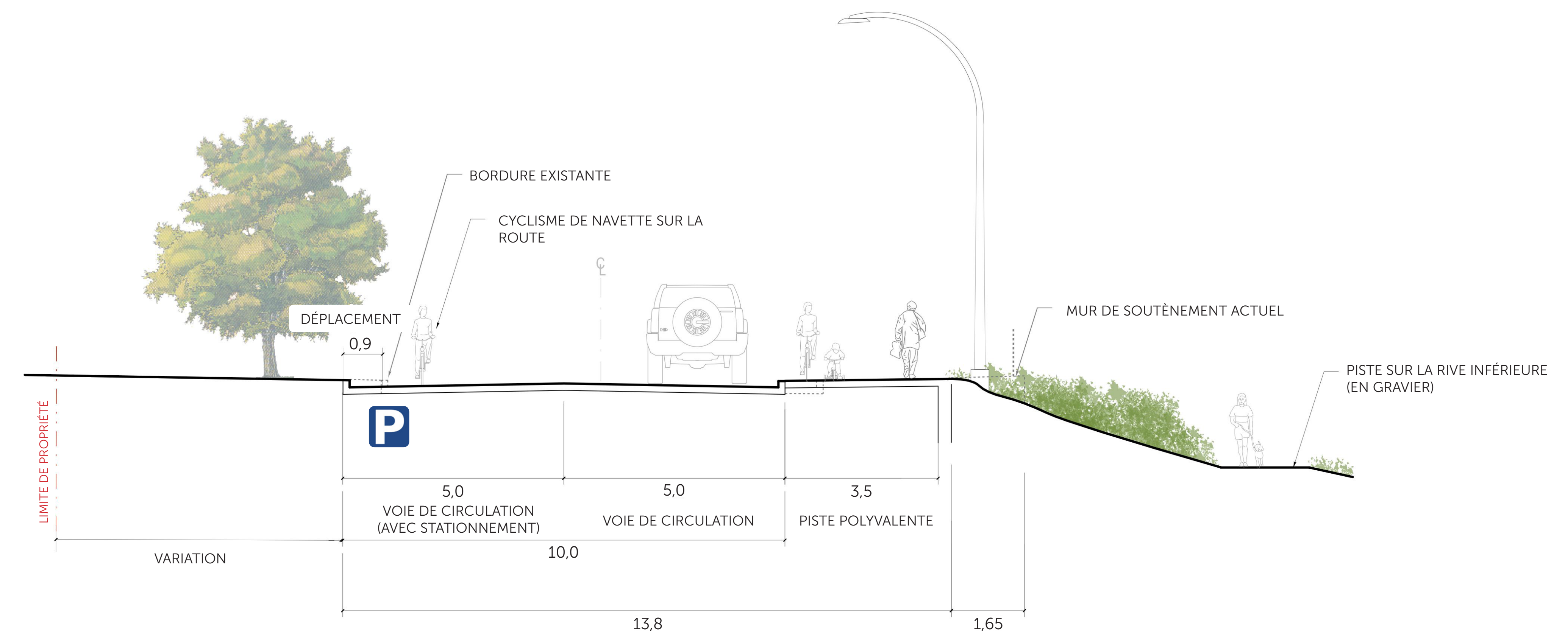
Section portant sur le concept proposé n° 2
