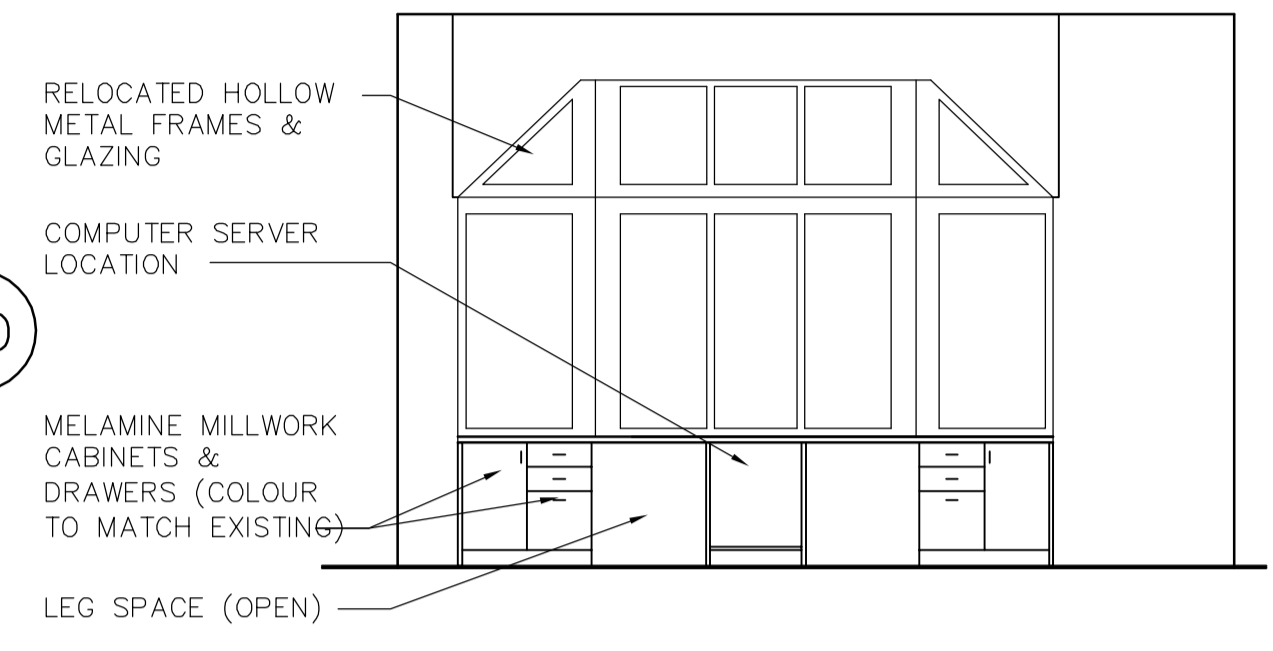
4 ELEVATION A1.01 1:50
