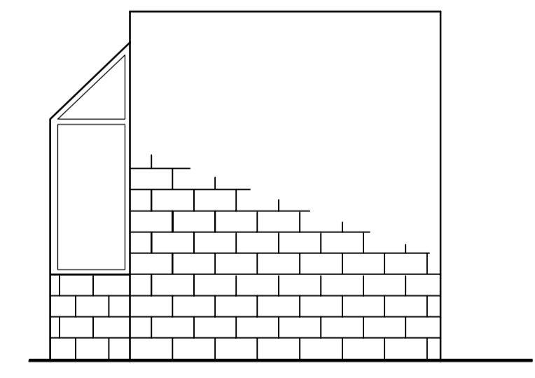
6 ELEVATION A1.01 1:50
