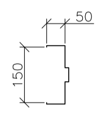
TYPE 1 FRAME TYPES SCALE: 1:10
