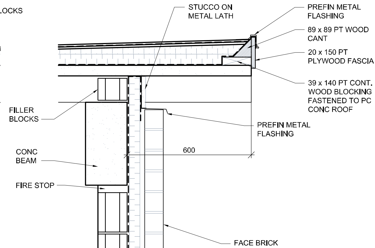
7 DETAIL SCALE: 1:10
