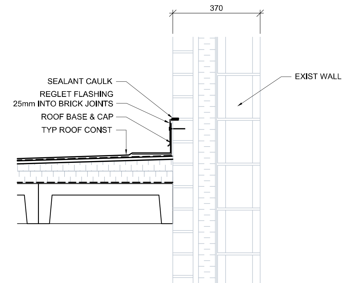
8 DETAIL SCALE: 1:10
