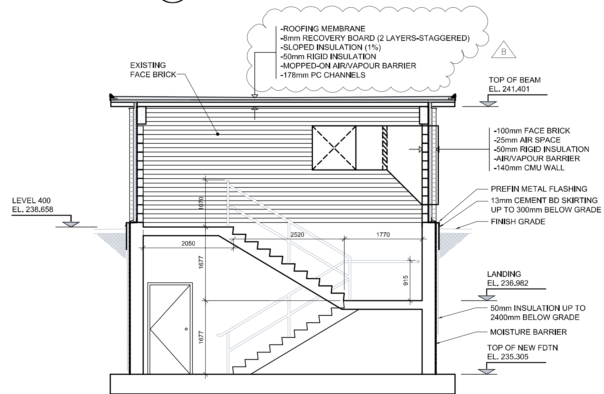
3 STAIR SECTION SCALE: 1:50
