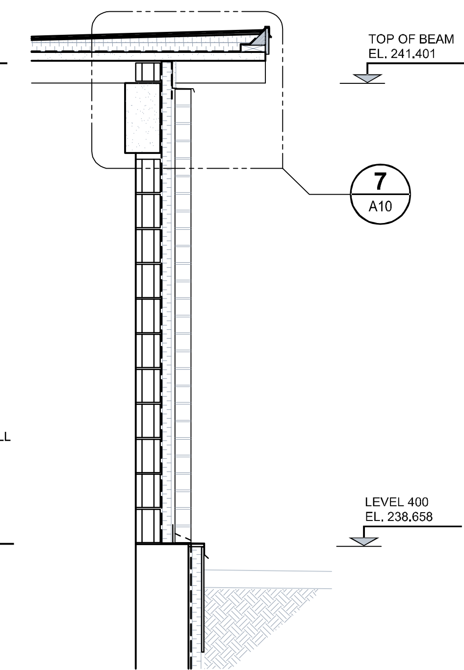
5 WALL SECTION SCALE: 1:20
