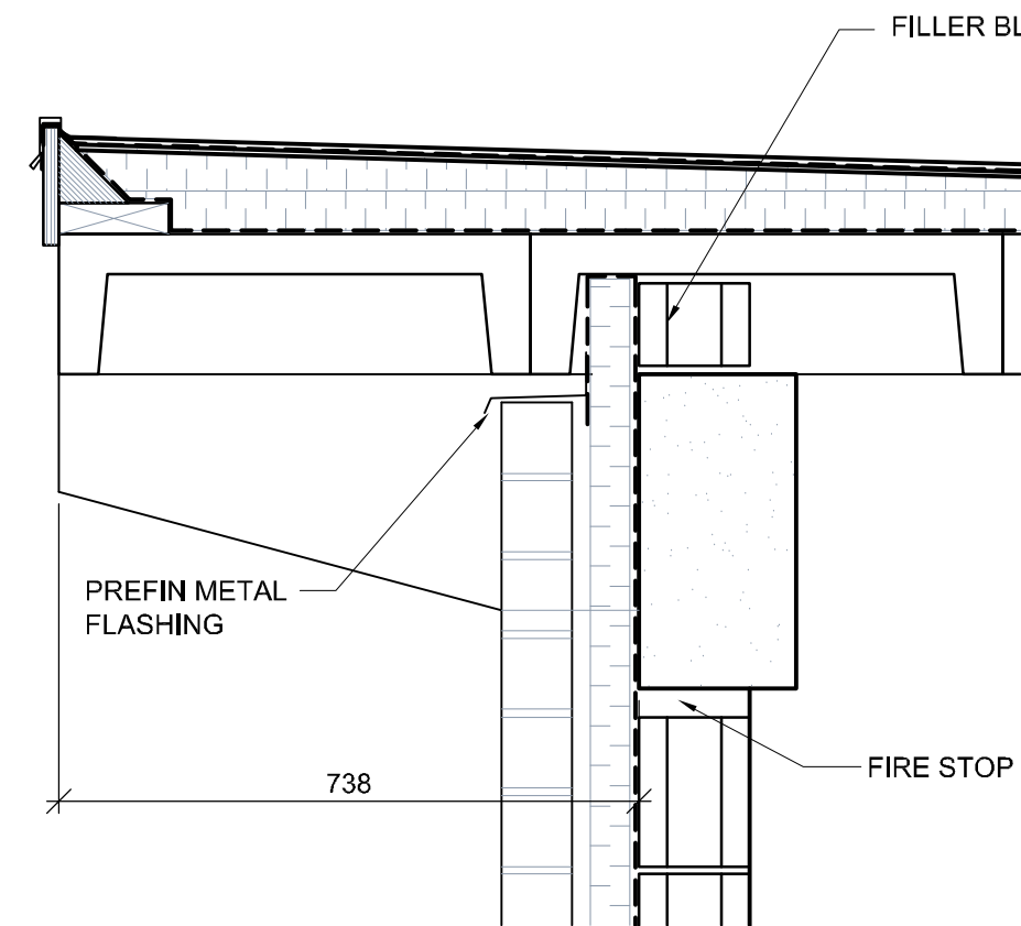
6 DETAIL SCALE: 1:10
