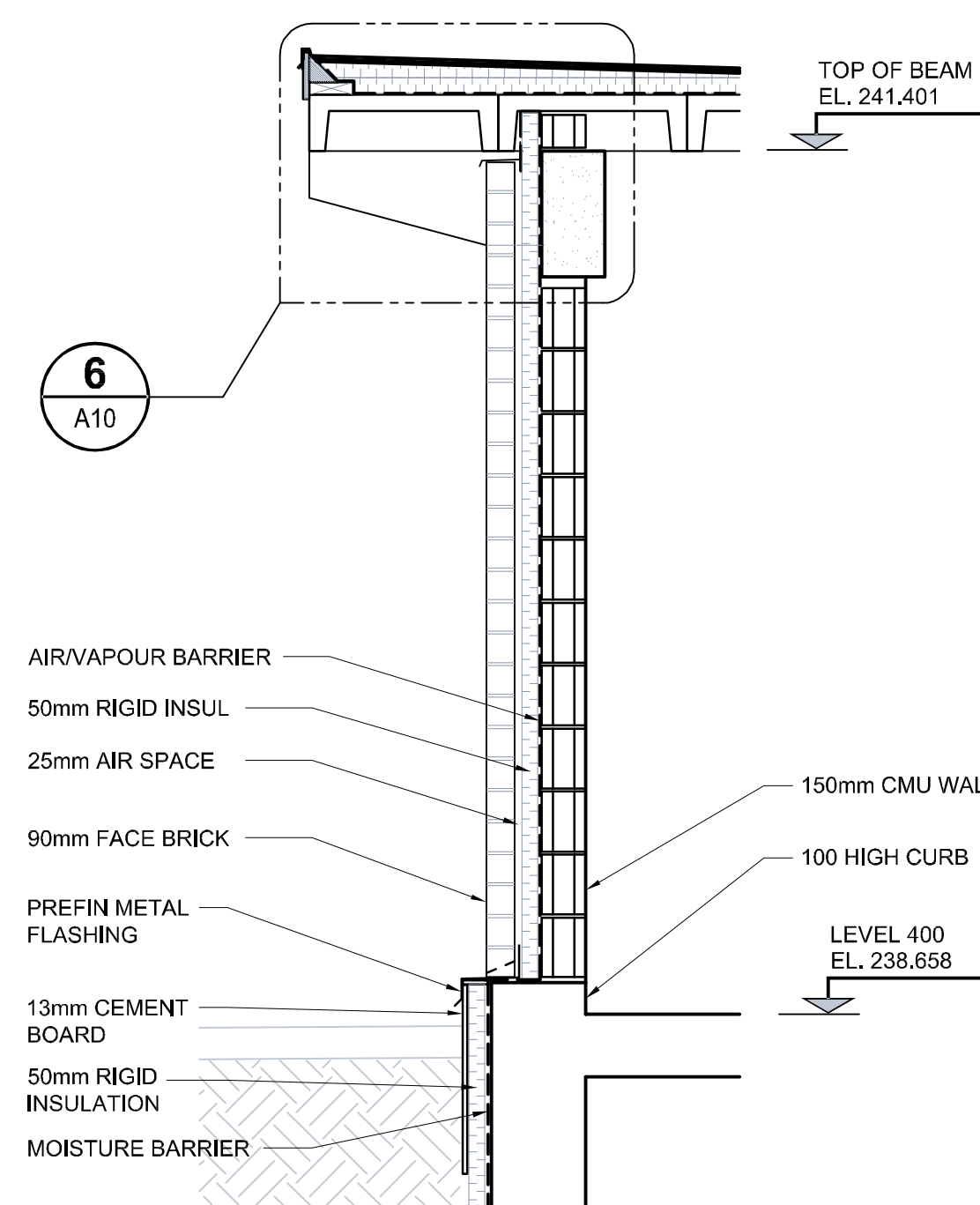
4 WALL SECTION SCALE: 1:20
