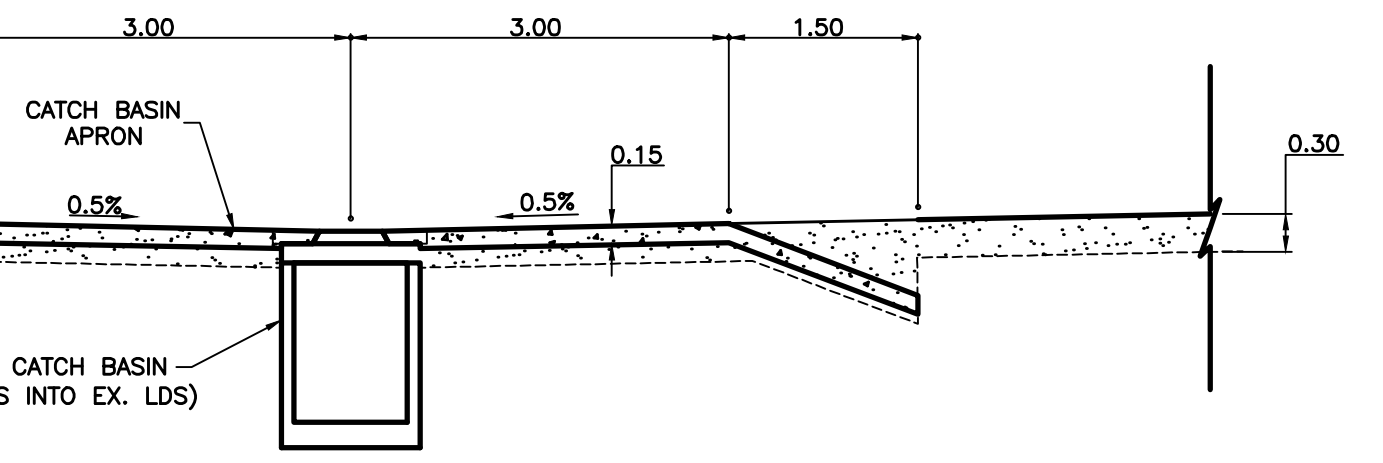
2 Catch Basin Apron N.T.S.
