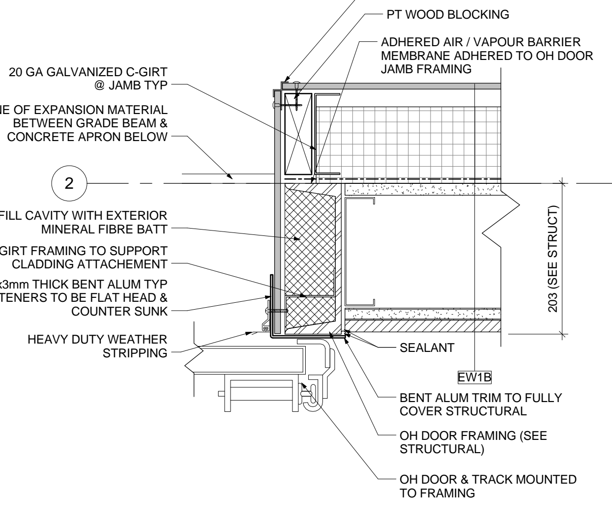
3 OVERHEAD DOOR JAMB 1:5
