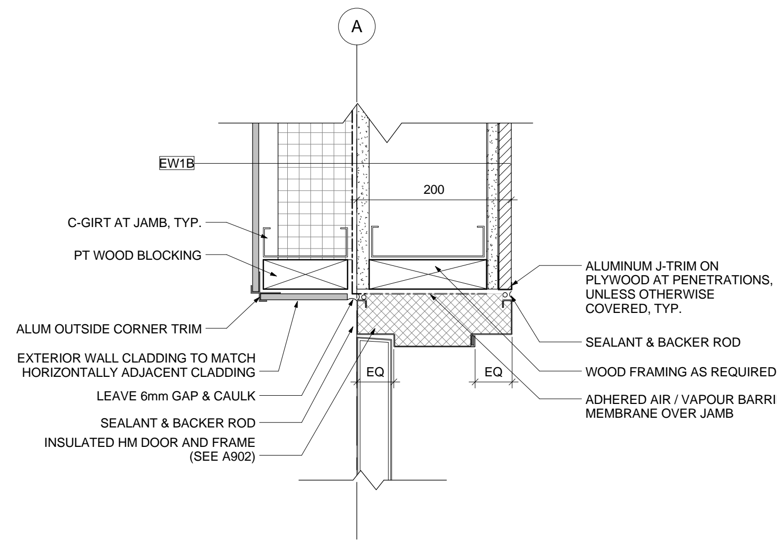
1 DOOR JAMB @ STEEL STUD INFILL 1:5
