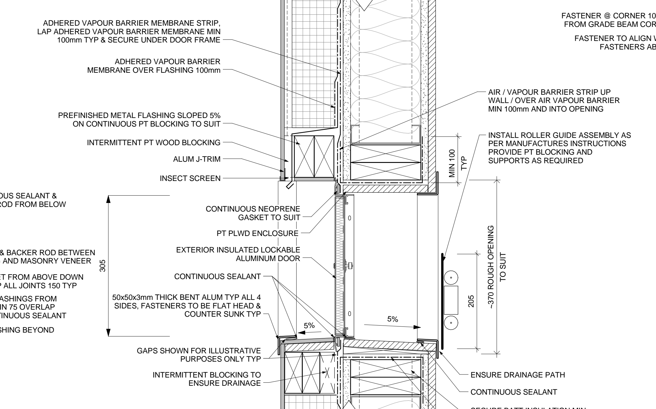
10 SECTION DETAIL - HOSE DOOR 1:5
