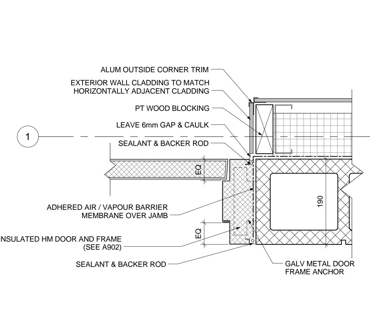
2 DOOR JAMB @ BLOCK INFILL 1:5
