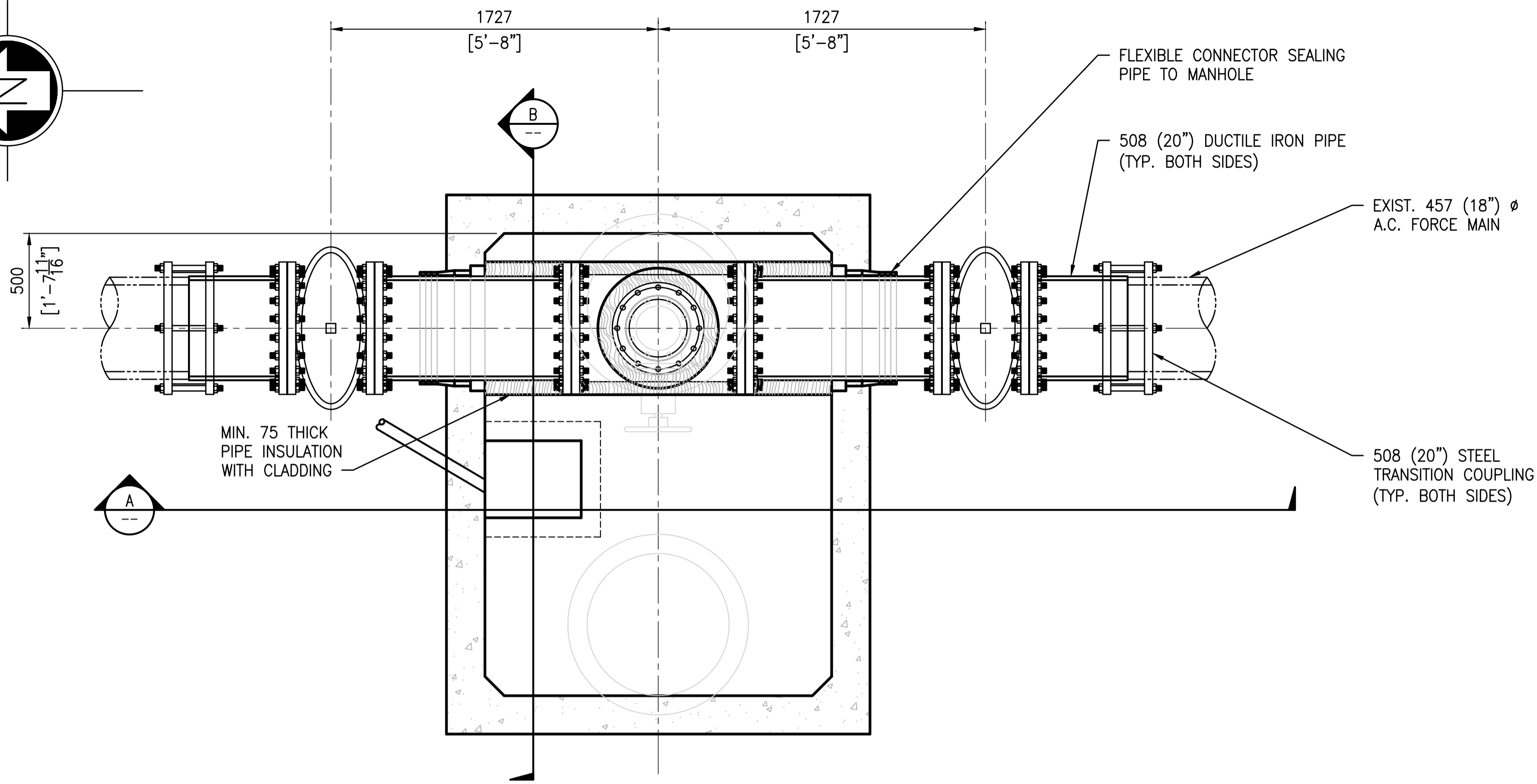
PLAN SCALE: 1 : 20
