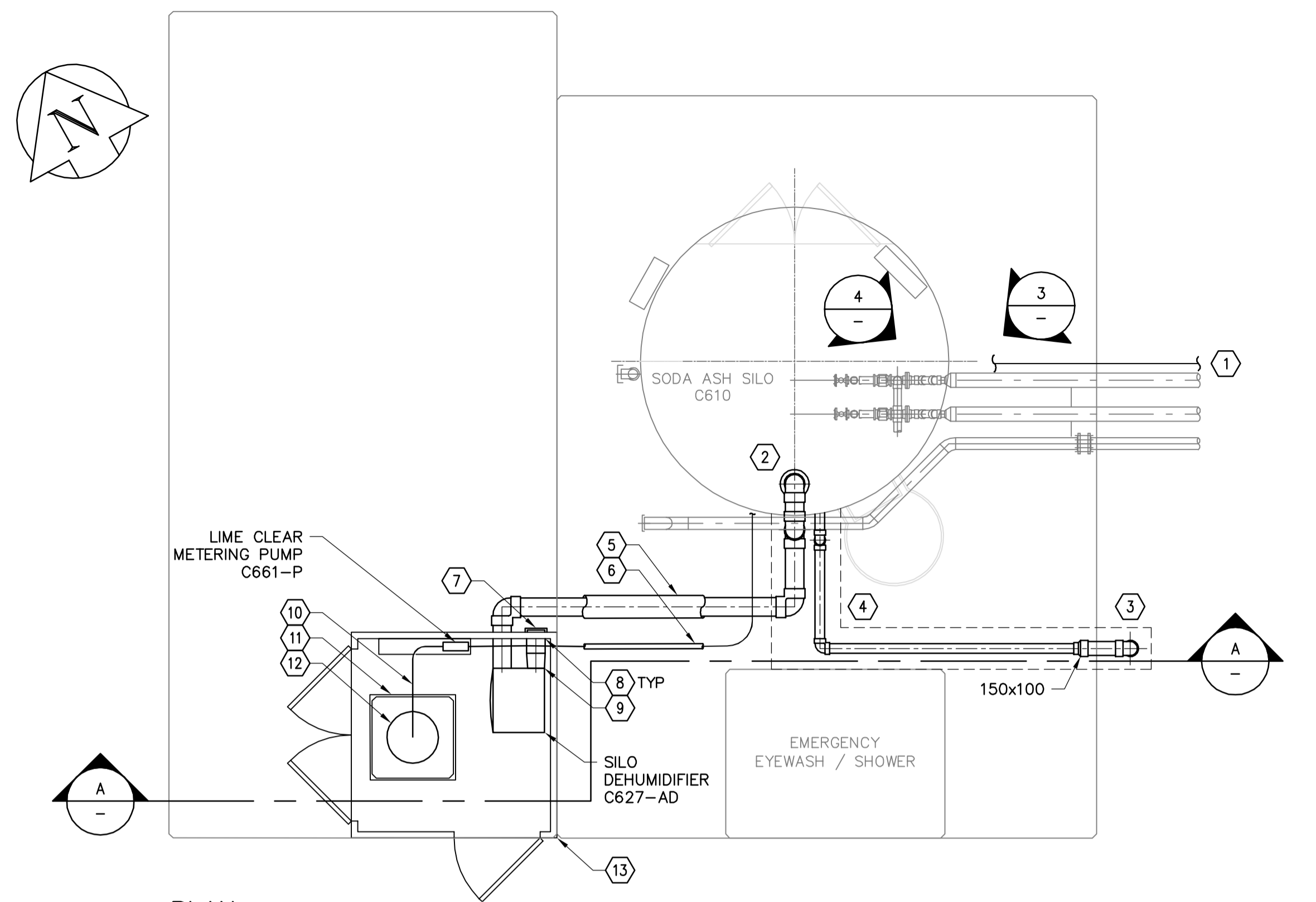
PLAN SCALE : 1:50
