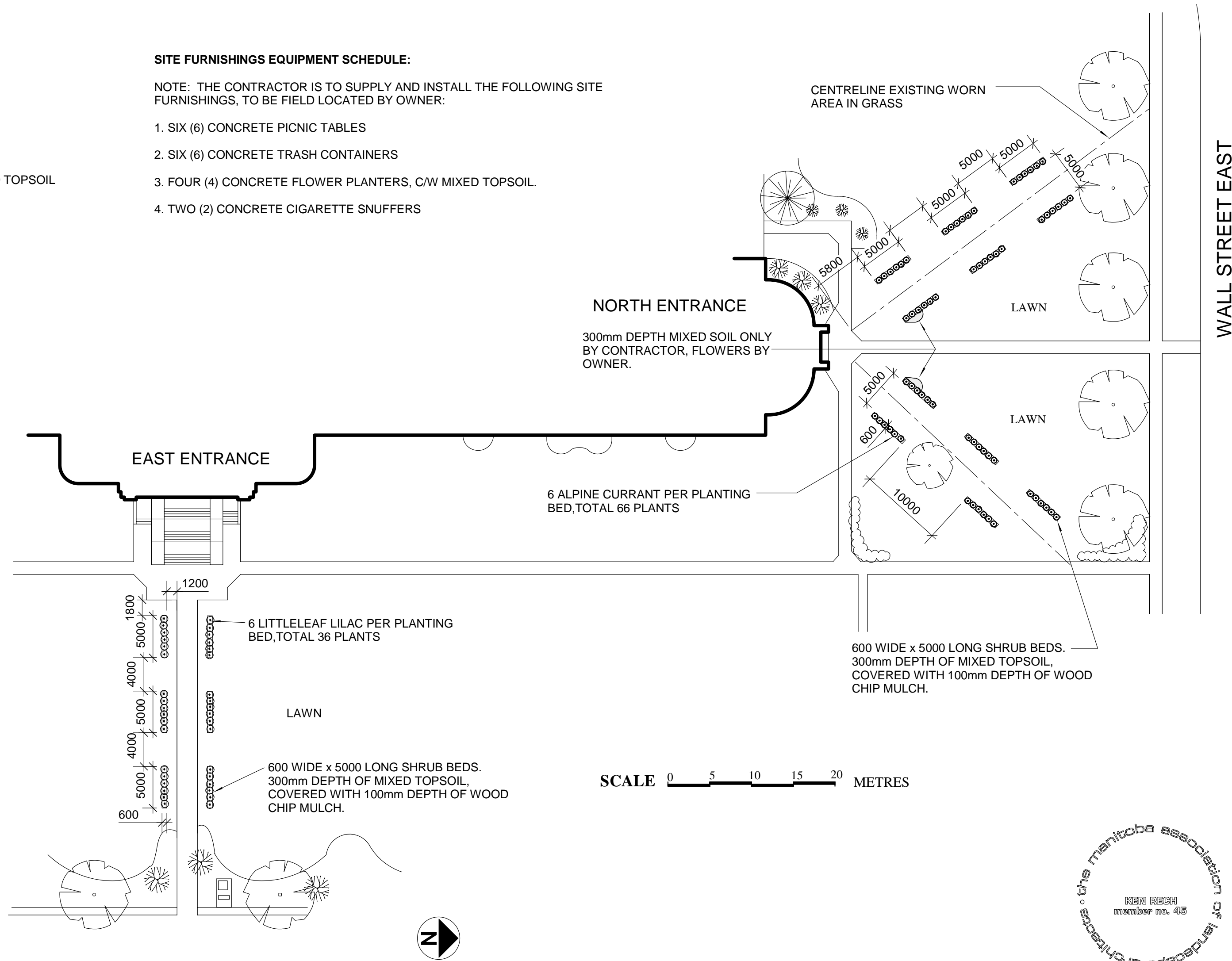
1 LANDSCAPE PLAN L6 Scale: 1:400
