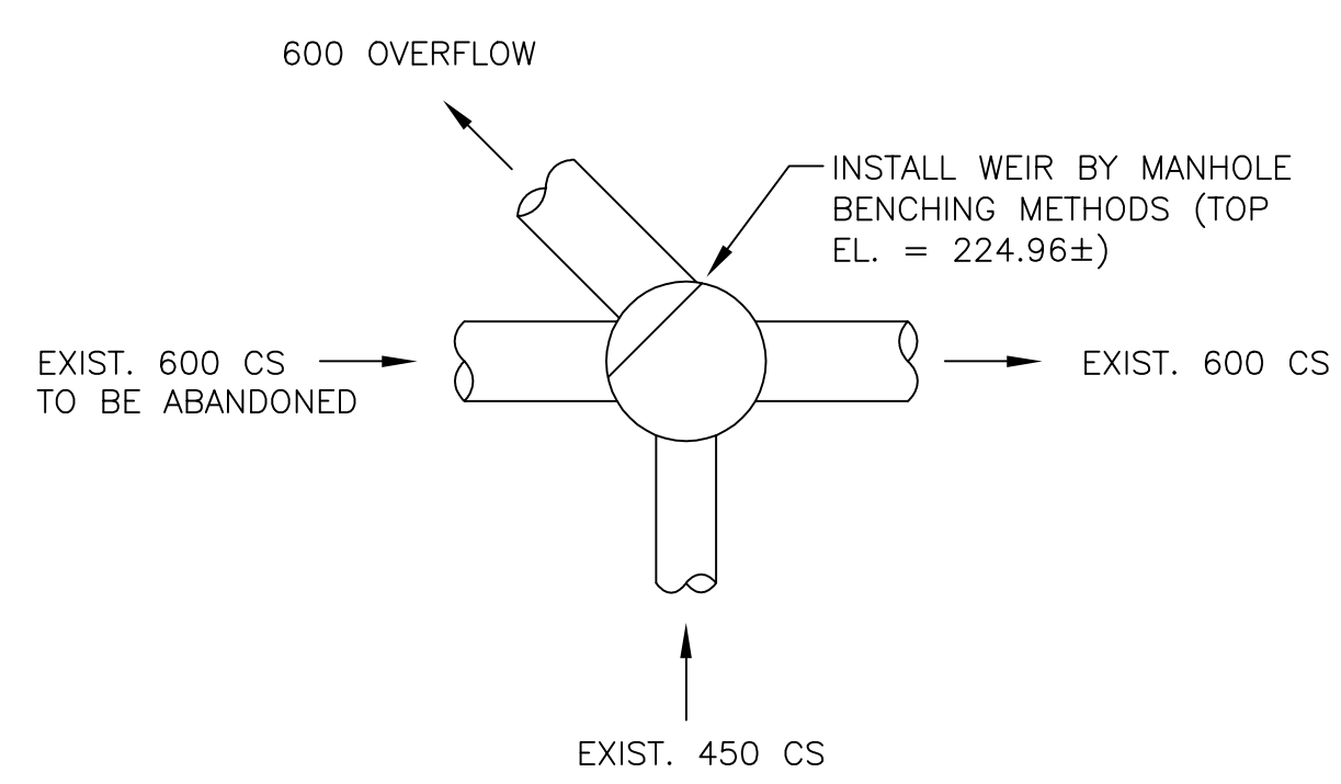
OVERFLOW DETAIL N.T.S.
