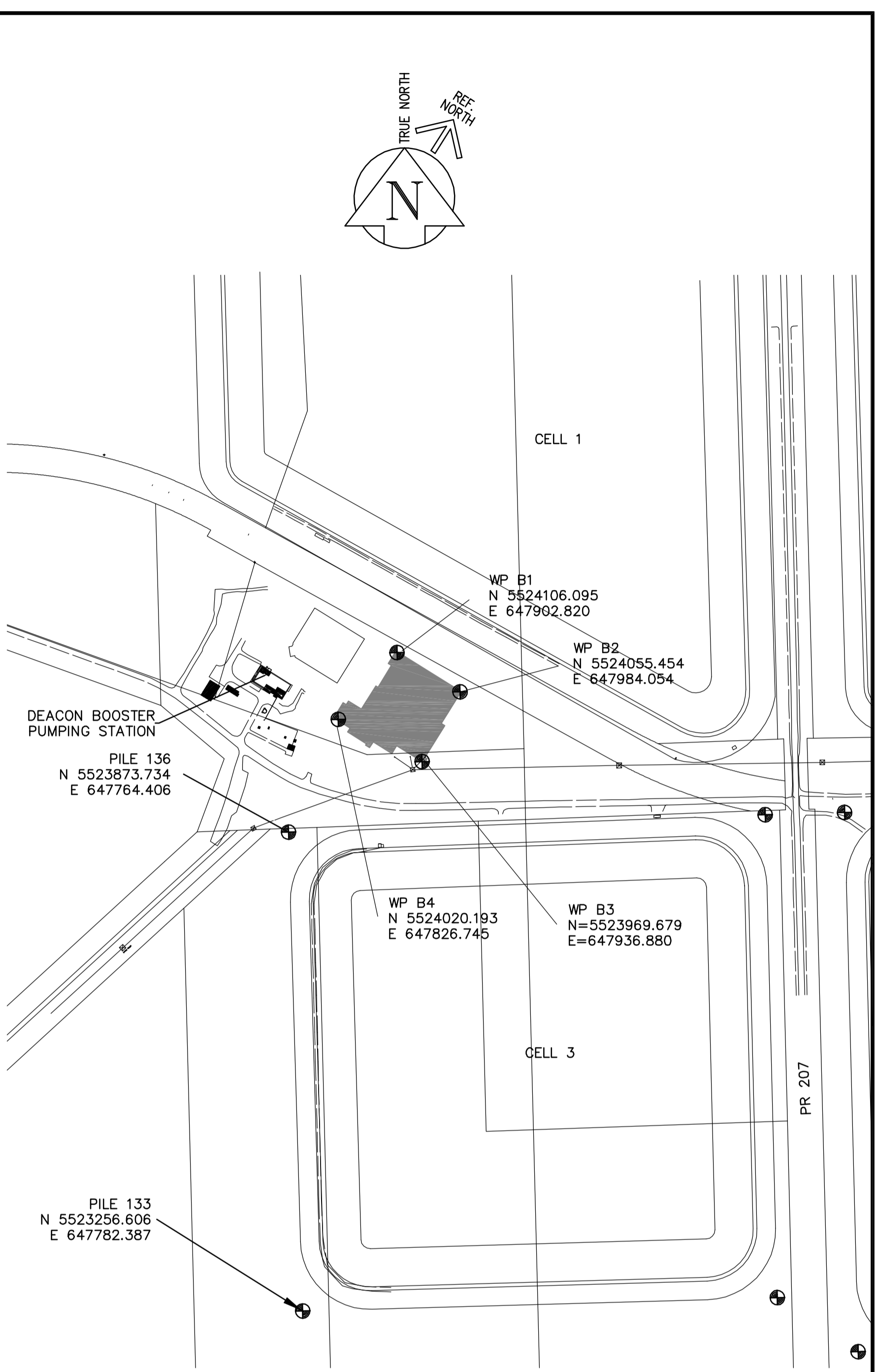
SURVEY PLAN N.T.S.
