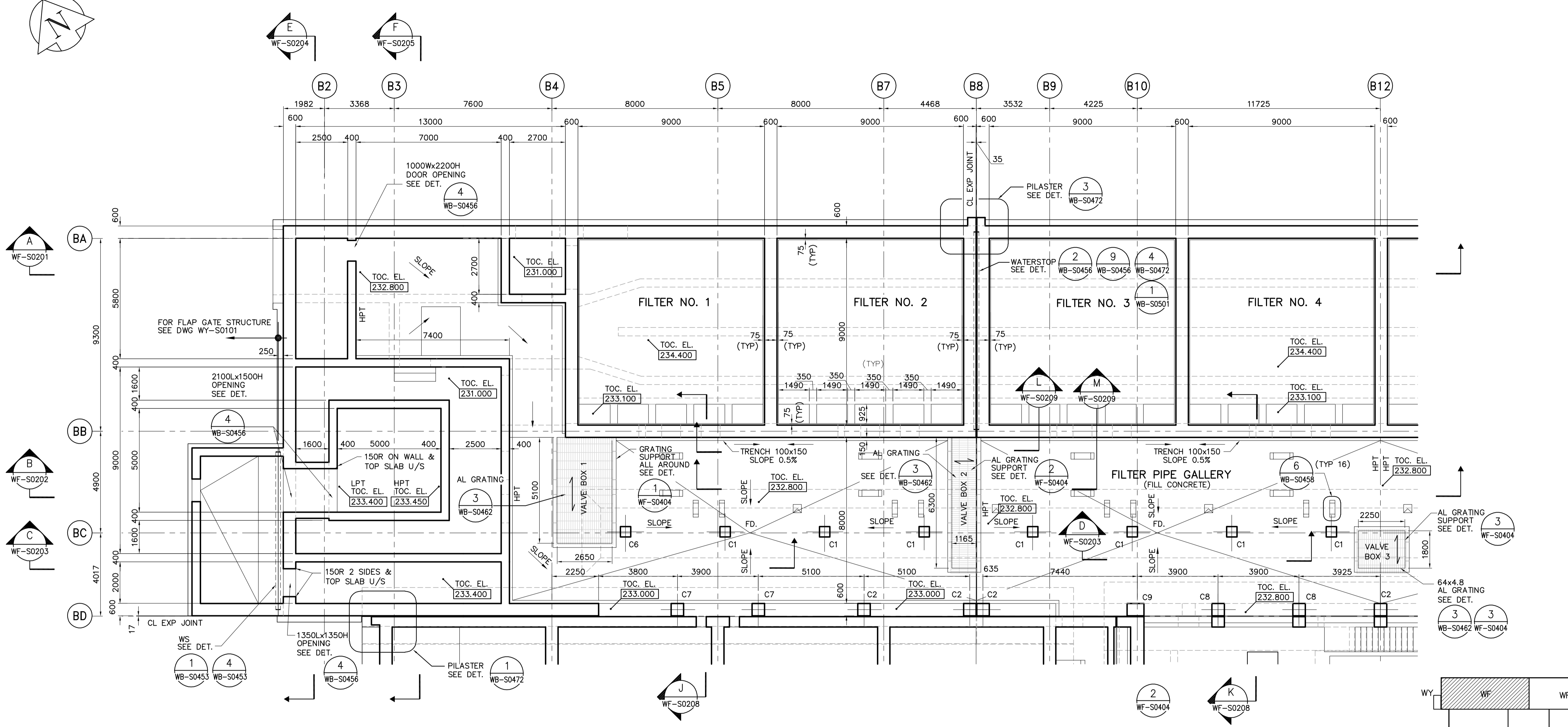
PLAN AT EL 234.400 1:100
