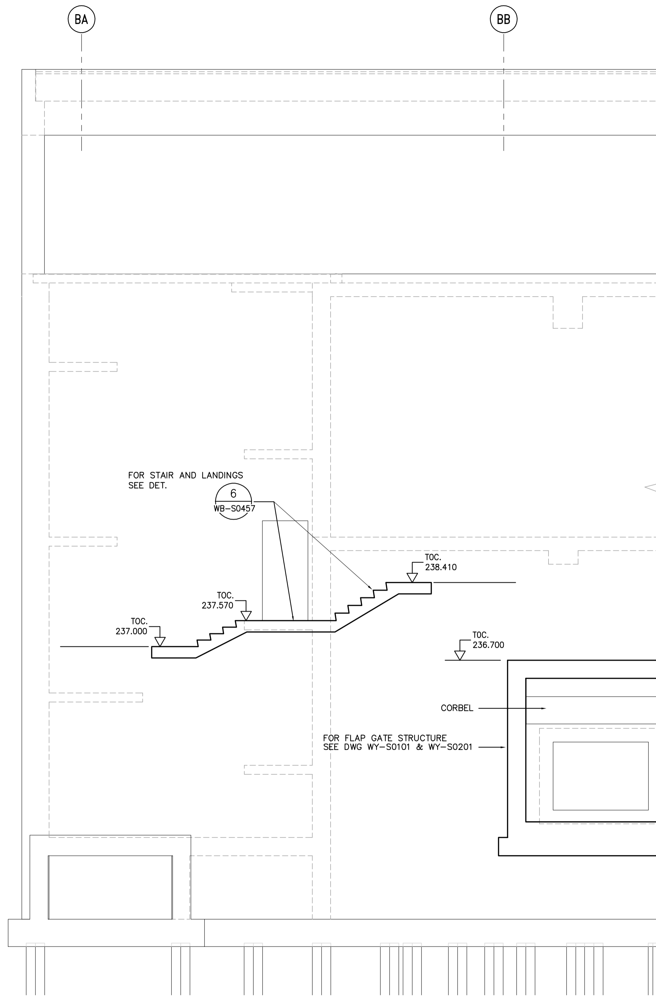
0 SECTION WF-S0101 1:50
