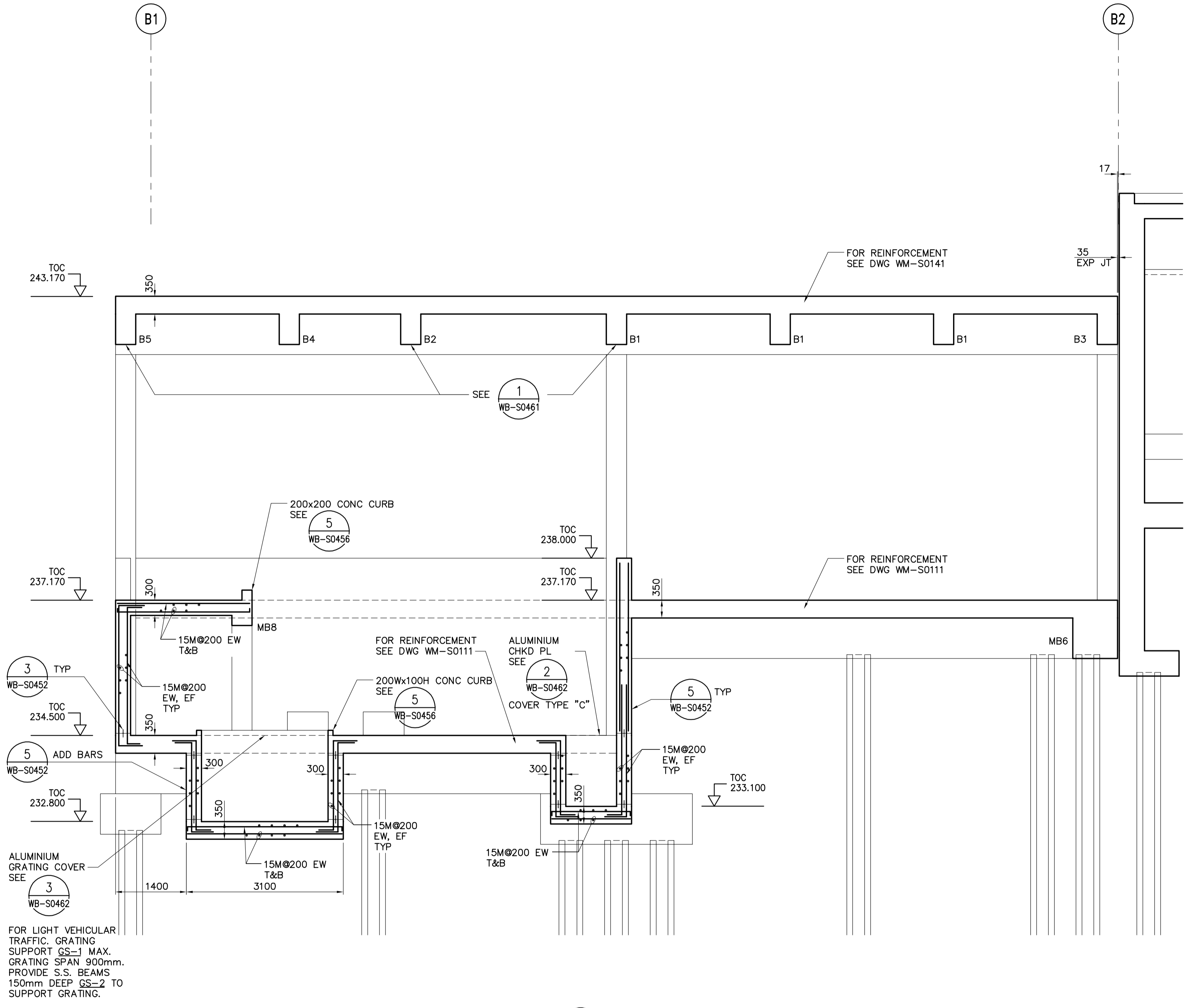
F SECTION WM-F0105 1:50 WM-S0111 WM-S0141 WM-S0146
