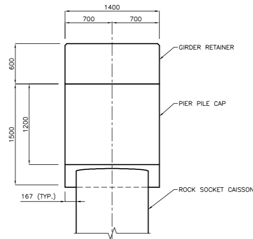
PIER SECTION B 1:25
