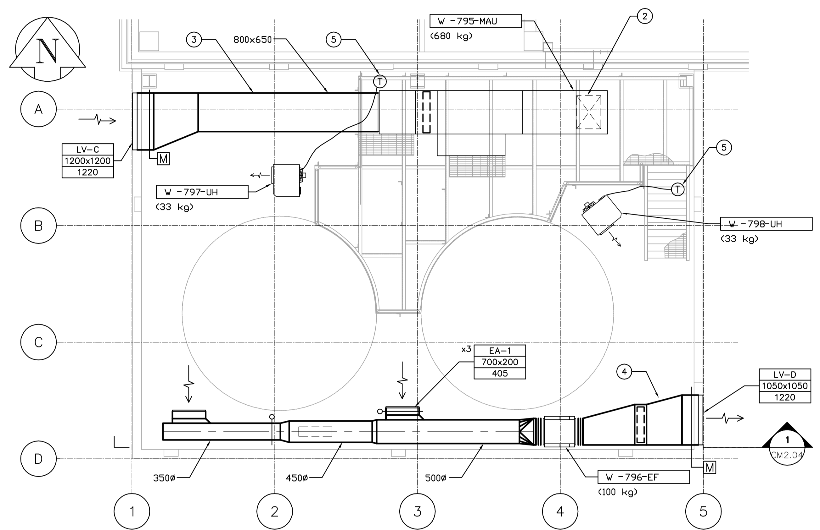
HVAC PLAN - MEZZANINE LEVEL SCALE: 1:50
