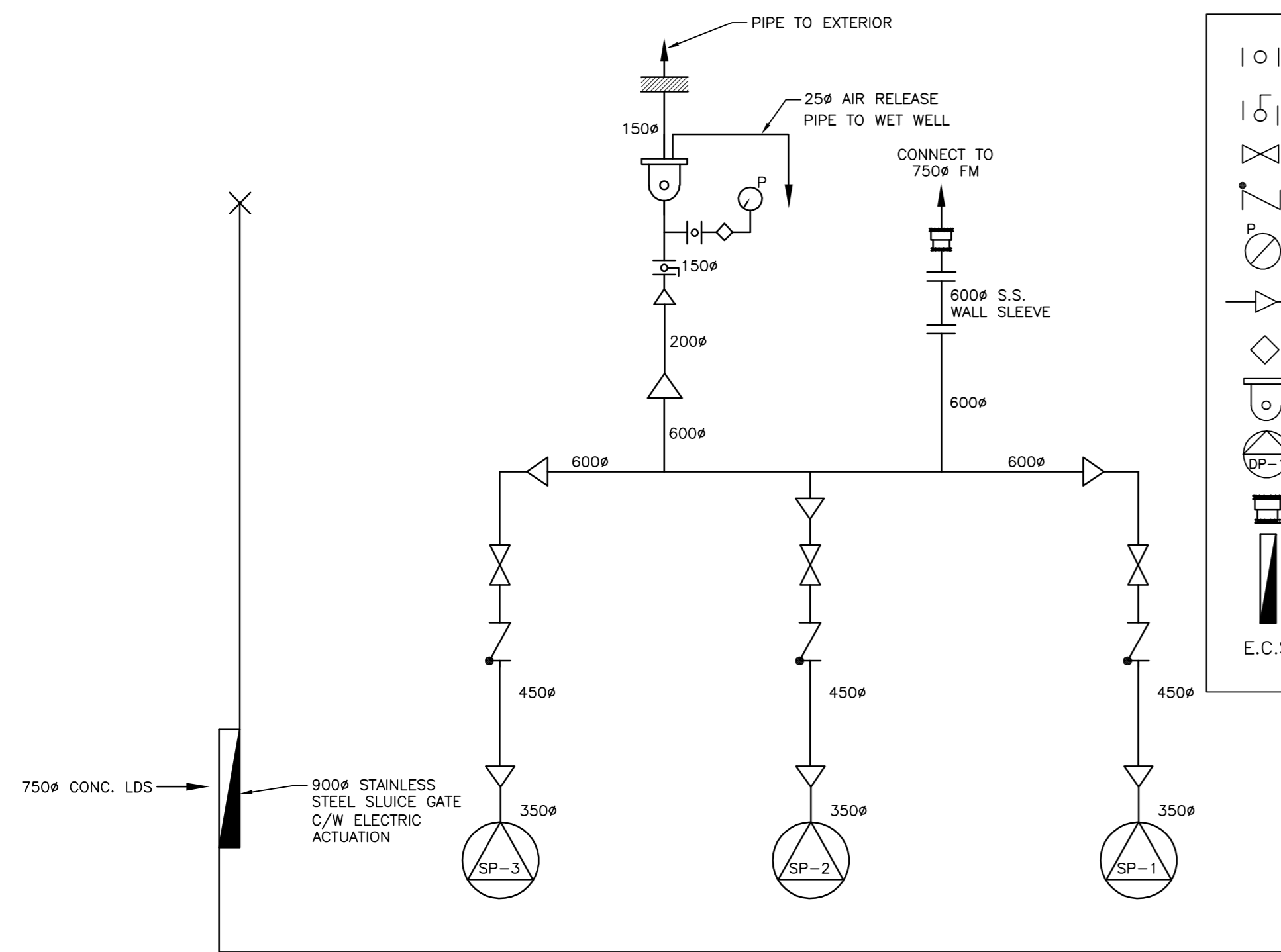
PROCESS SCHEMATIC N.T.S.
