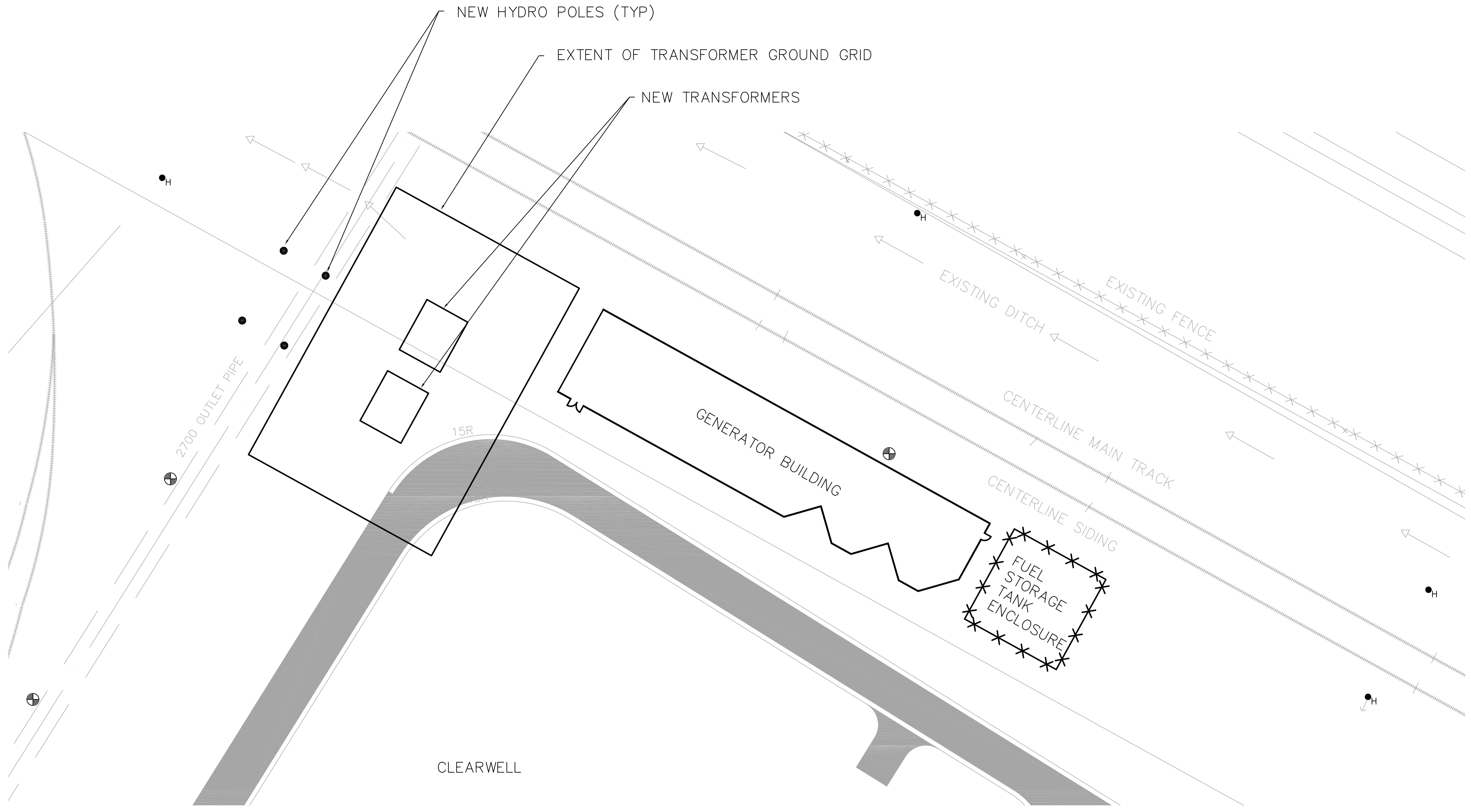
SITE PLAN SCALE: 1:250
