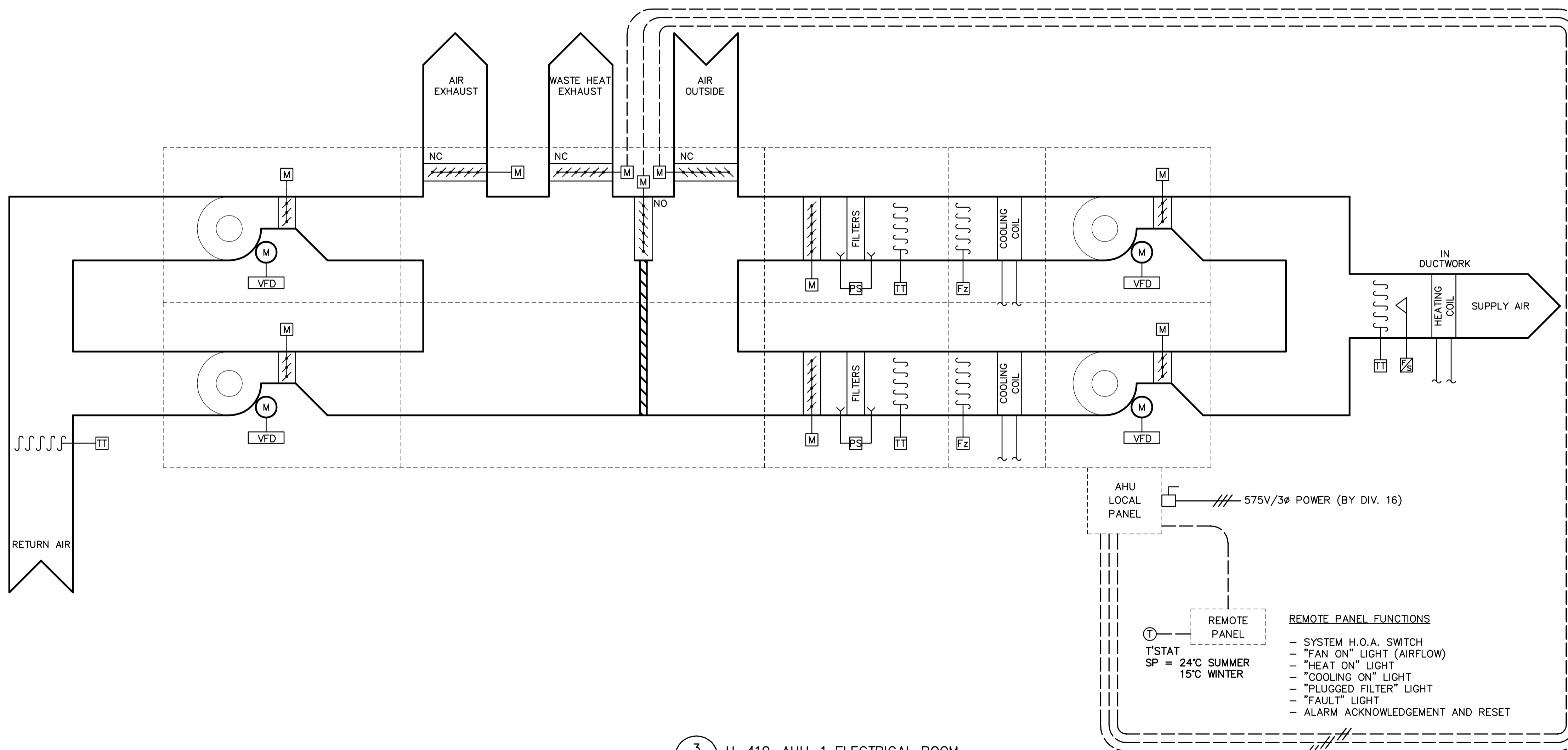
3 U-410-AHU-1 ELECTRICAL ROOM M8.03 SCALE N.T.S.
