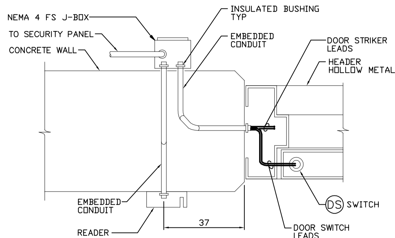
2 DETAIL DOOR JAMB NTS
