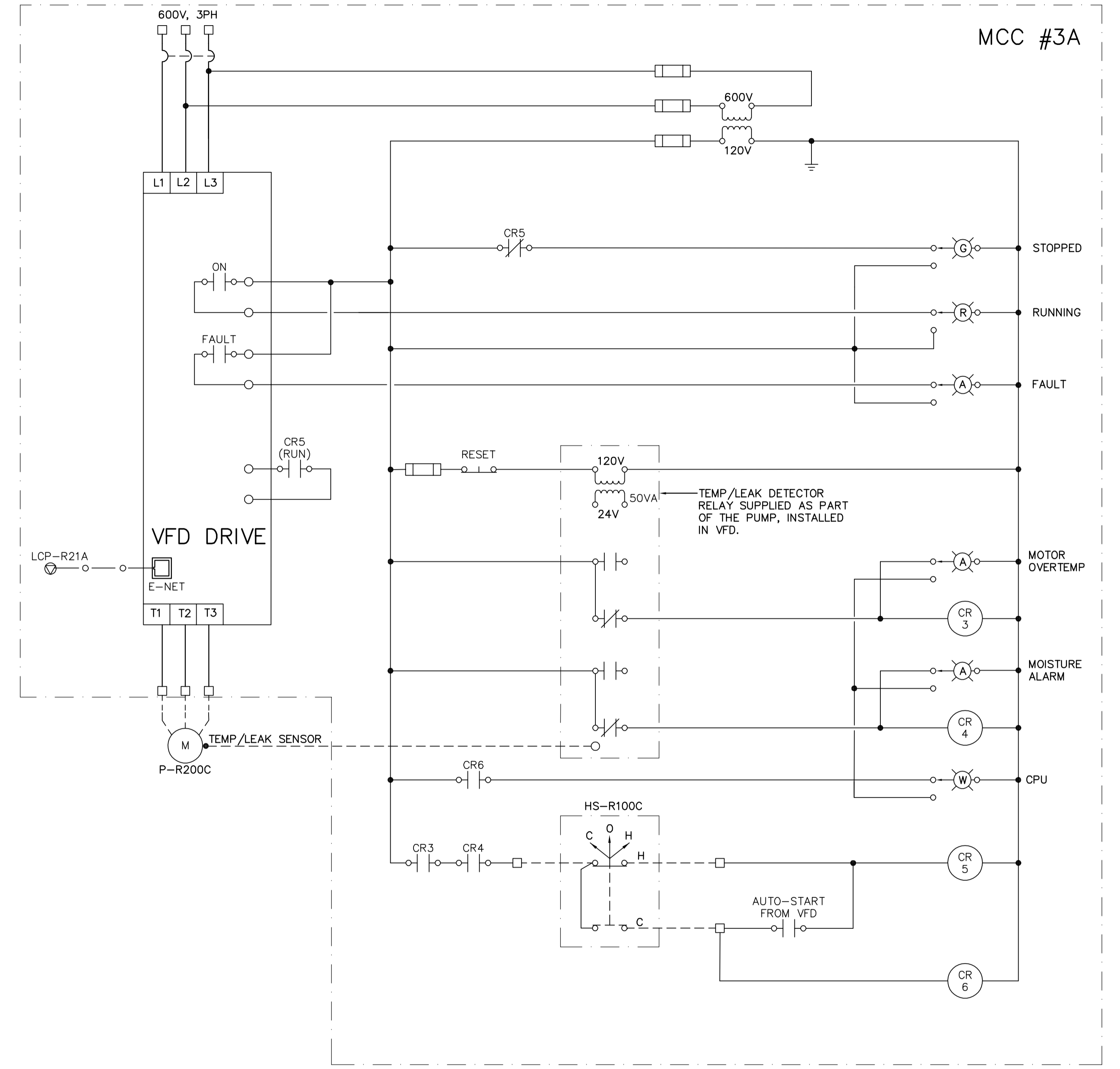
SLUDGE PUMP (P-R200C)
