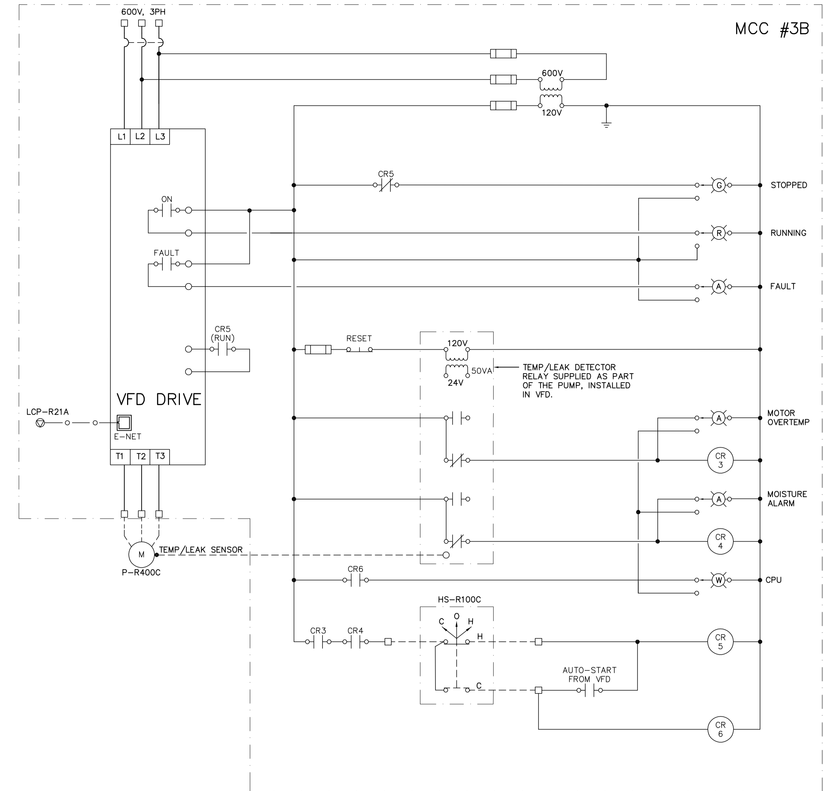
SLUDGE PUMP (P-R400C)
