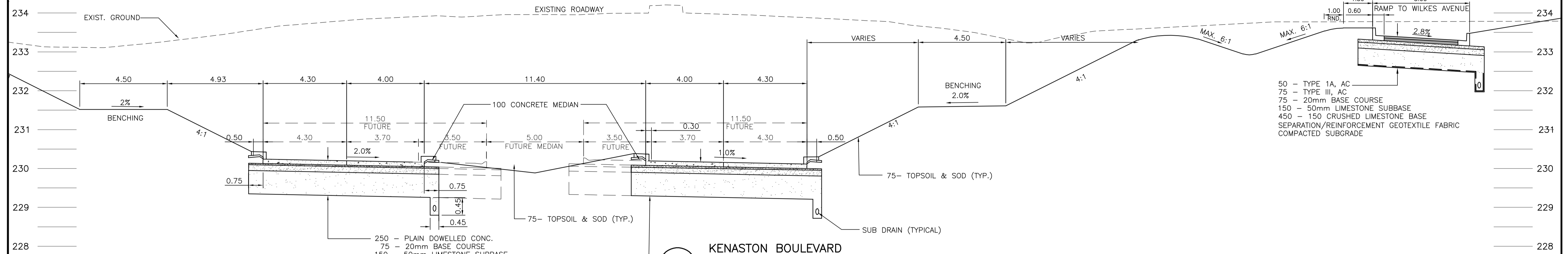
D KENASTON BOULEVARD SECTION @ STA 1+425 SCALE: HOR. 1:100 VERT. 1:50
