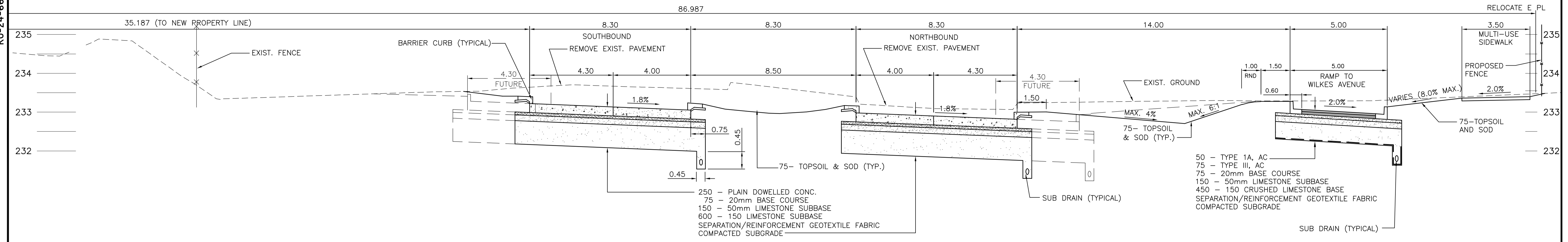
C KENASTON BOULEVARD SECTION @ STA 1+300 SCALE: HOR. 1:100 VERT. 1:50
