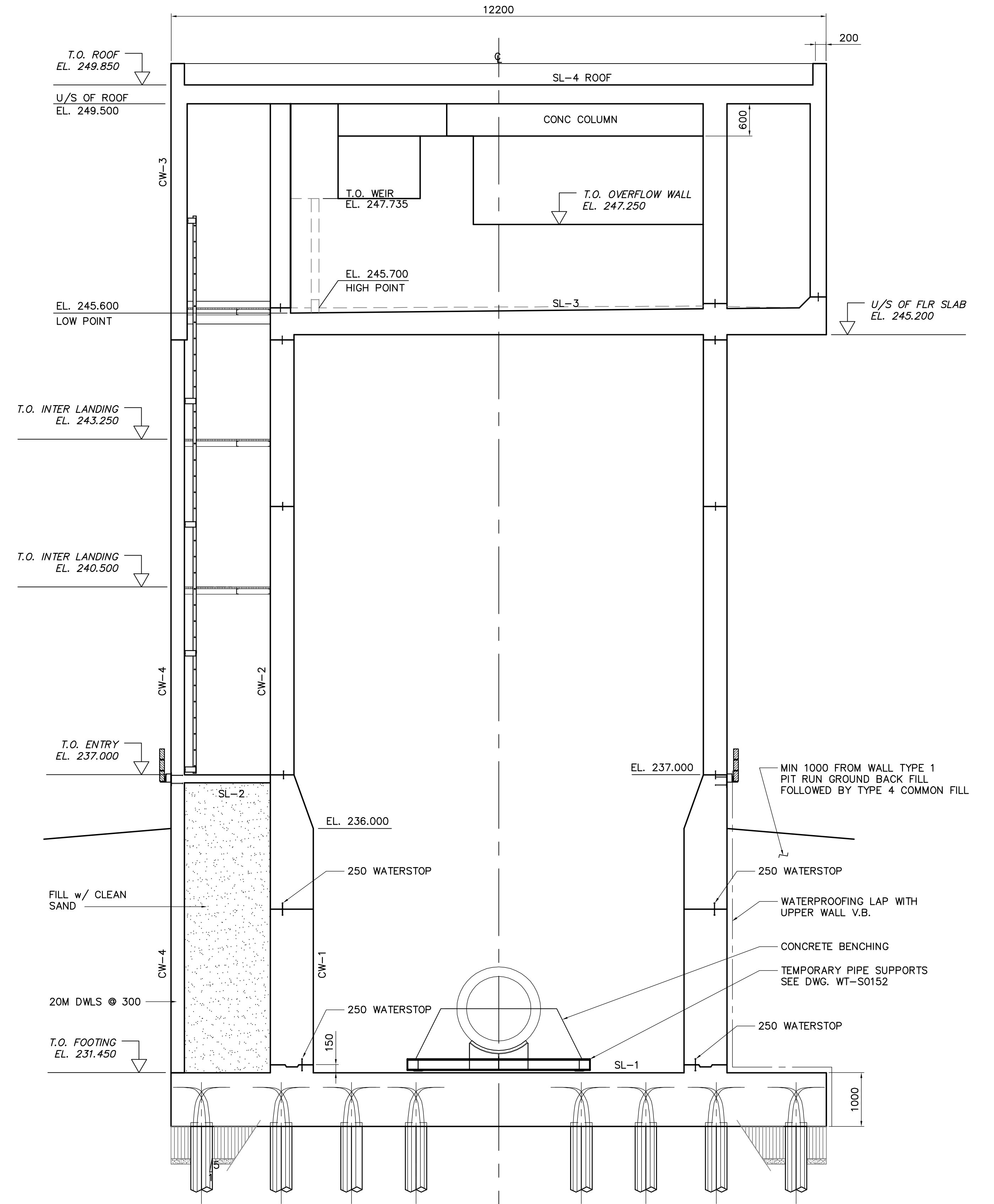
SECTION 2 WY-S0151 1:50
