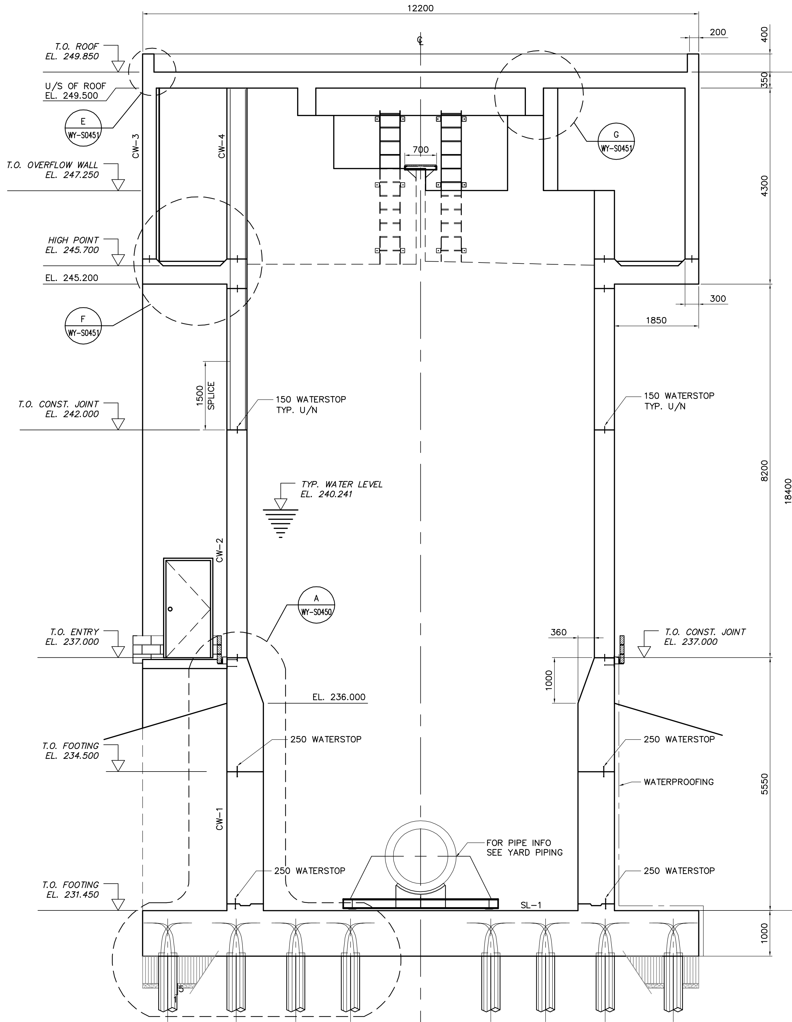
SECTION 1 WY-S0150/WY-S0151 1:50
