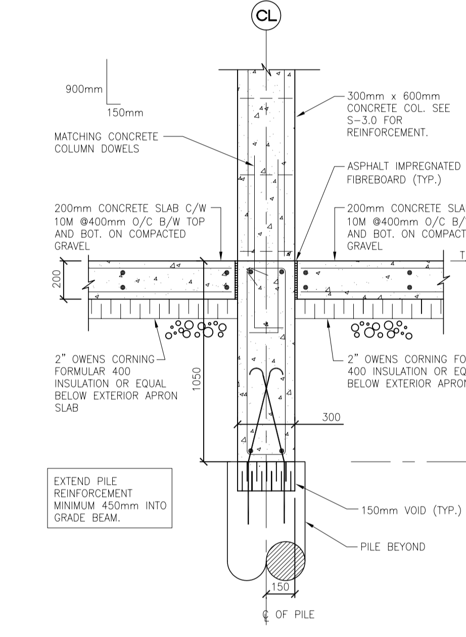
SECTION 8 SCALE: 120
