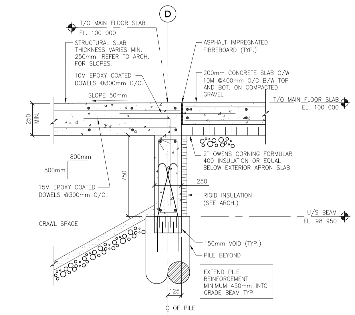
SECTION 6 SCALE: 120
