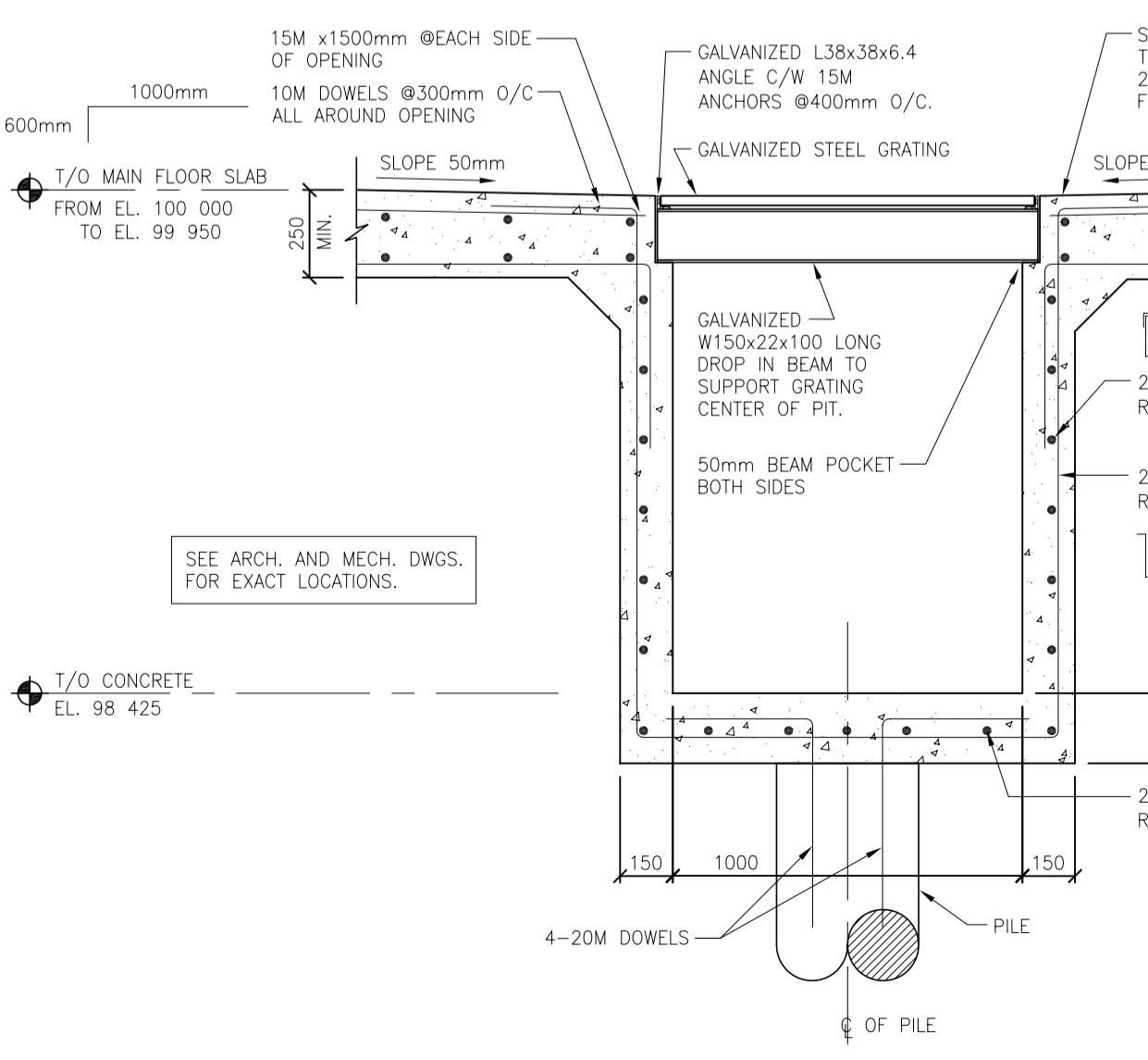
SECTION 11 SCALE: 120
