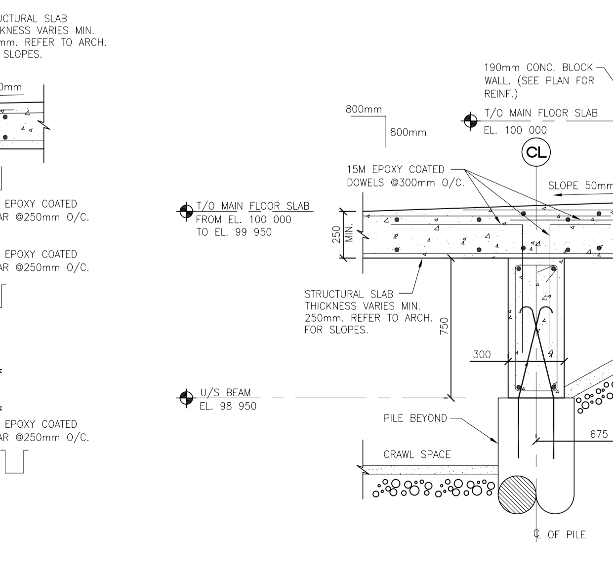
SECTION 12 SCALE: 120
