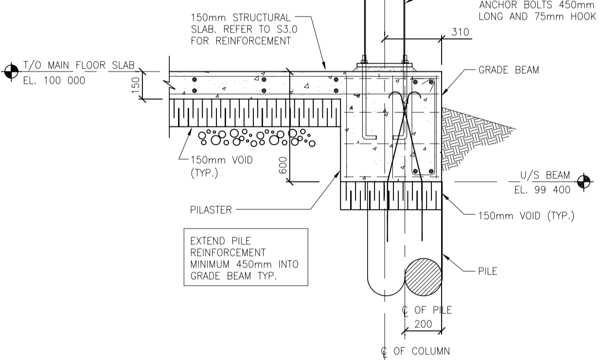
SECTION 10 SCALE: 120
