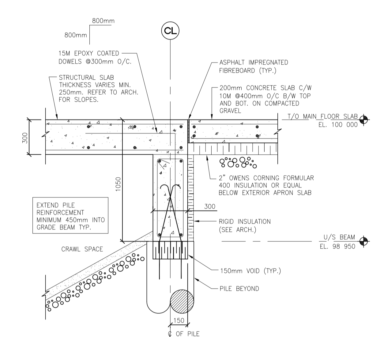
SECTION 7 SCALE: 120
