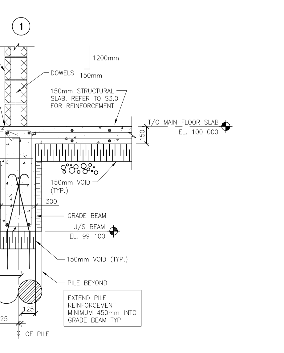
SECTION 12 SCALE: 120
