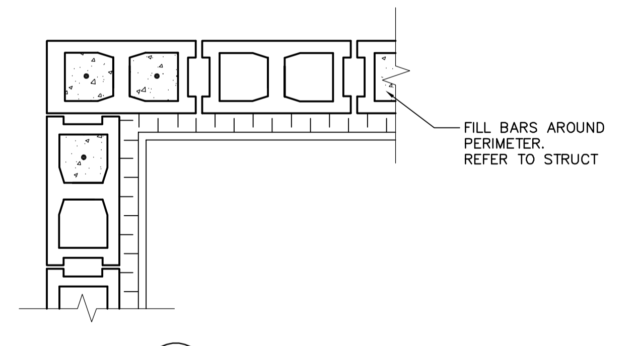
E DETAIL WY-S0160 1:10
