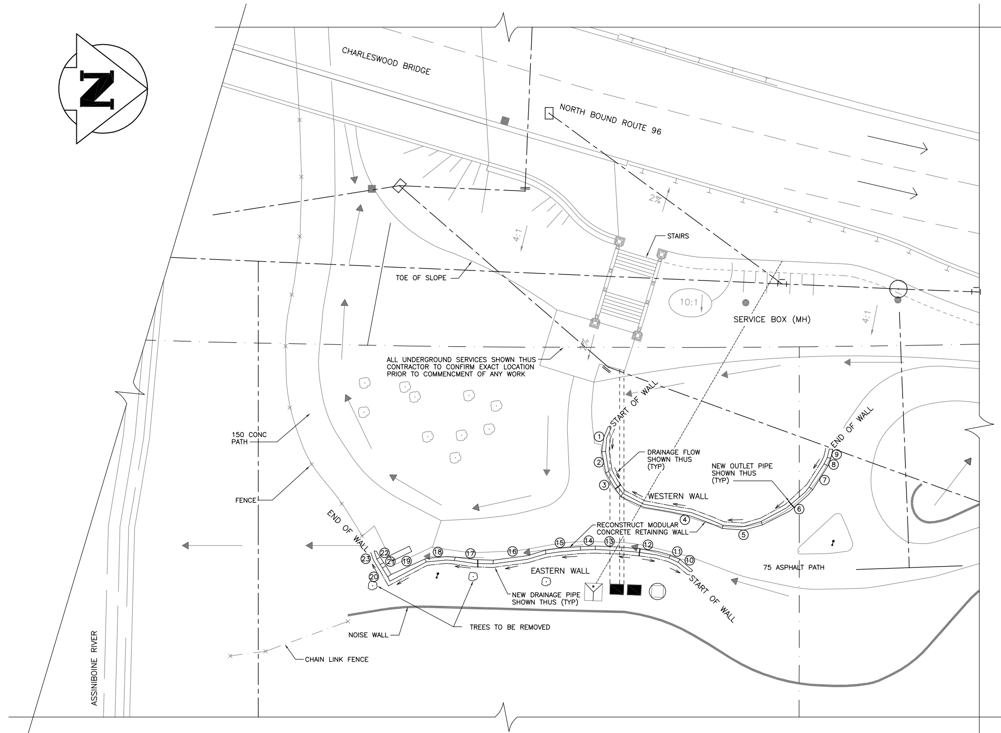
1 SITE PLAN 1 : 150
