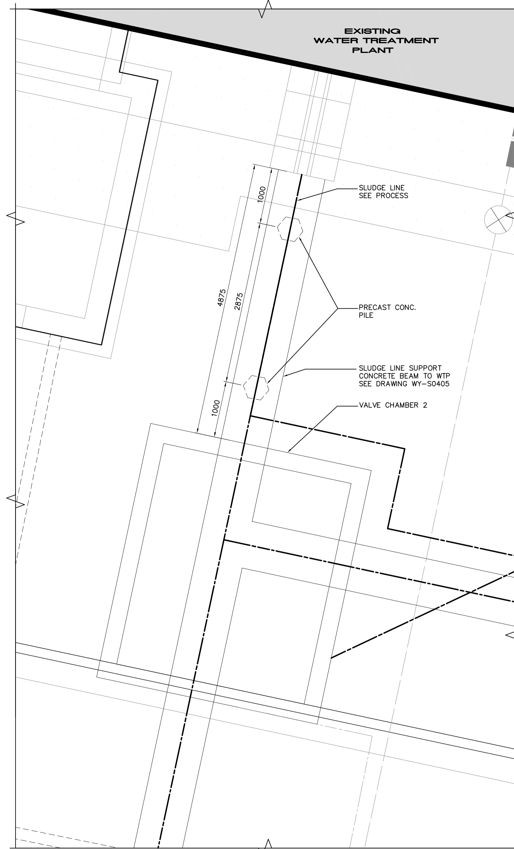
PLAN VIEW - PARTIAL N.T.S.
