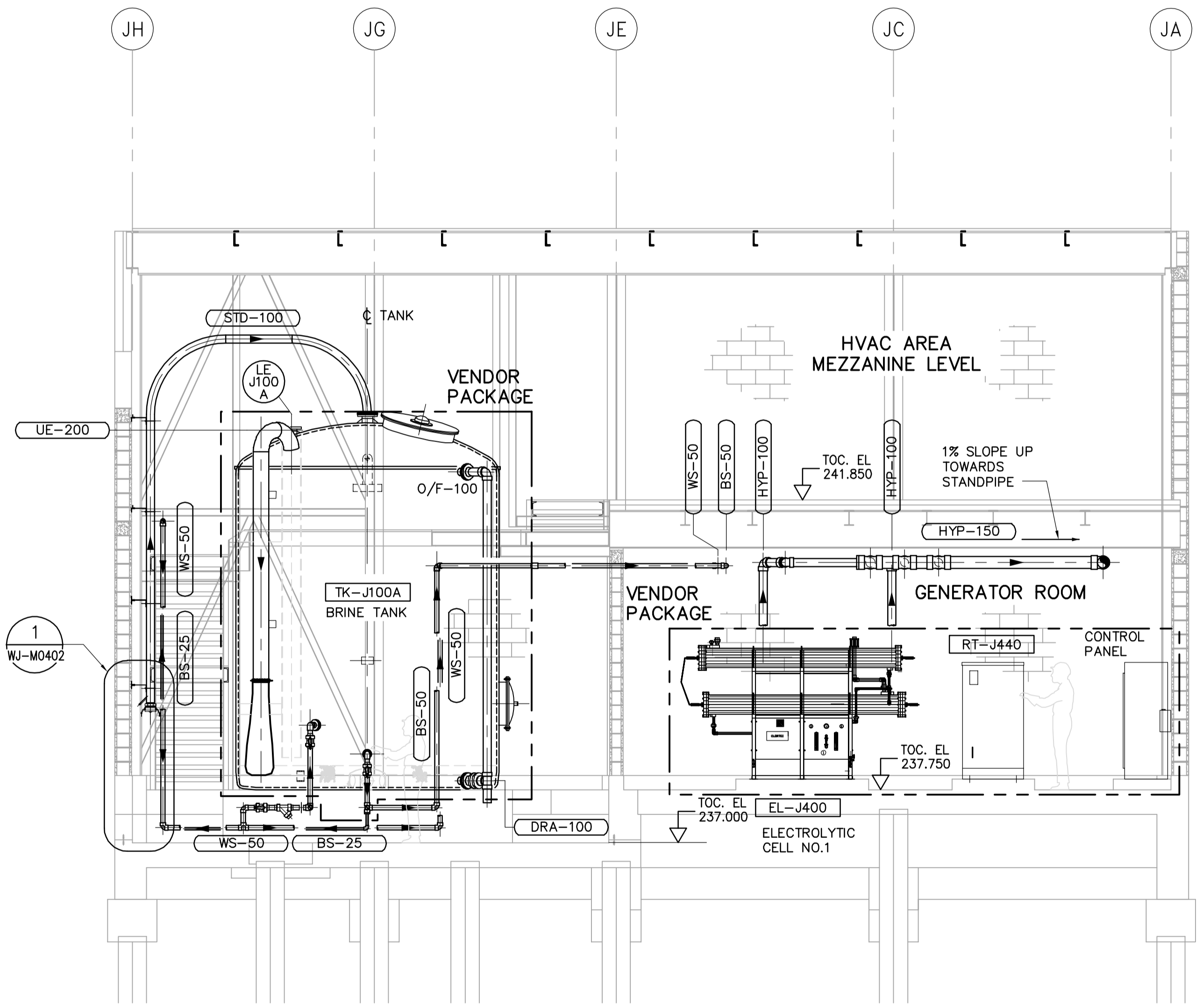
C SECTION WJ-M0111 1:50
