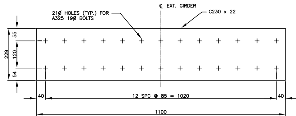
MK 1 - NEW C230 x 22 x 1100 N.T.S.
