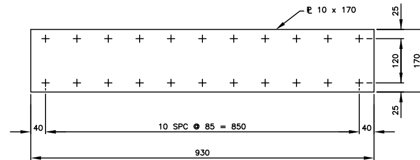
MK 4 - NEW P 10 x 70 x 930 N.T.S.
