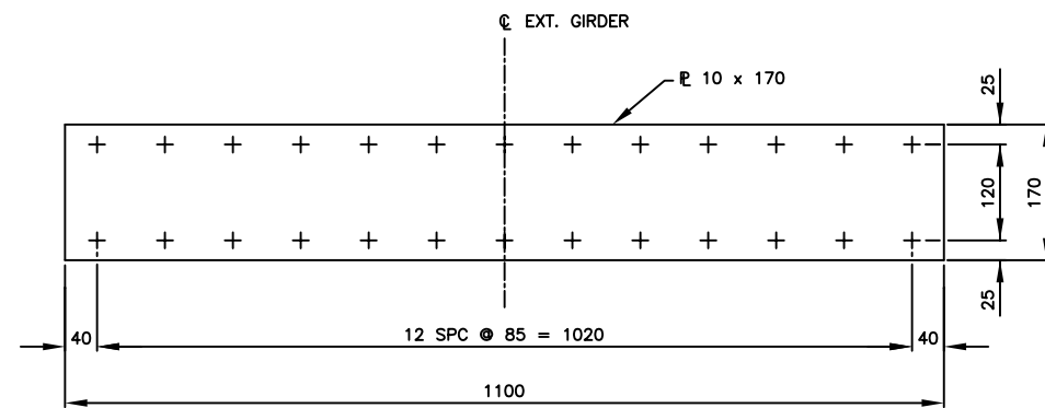
MK 2 - NEW P 10 x 70 x 1100 N.T.S.
