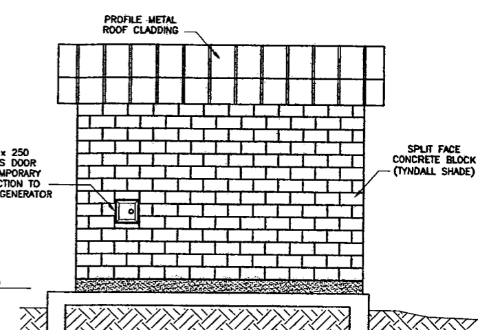
EAST ELEVATION SCALE: 1:40
