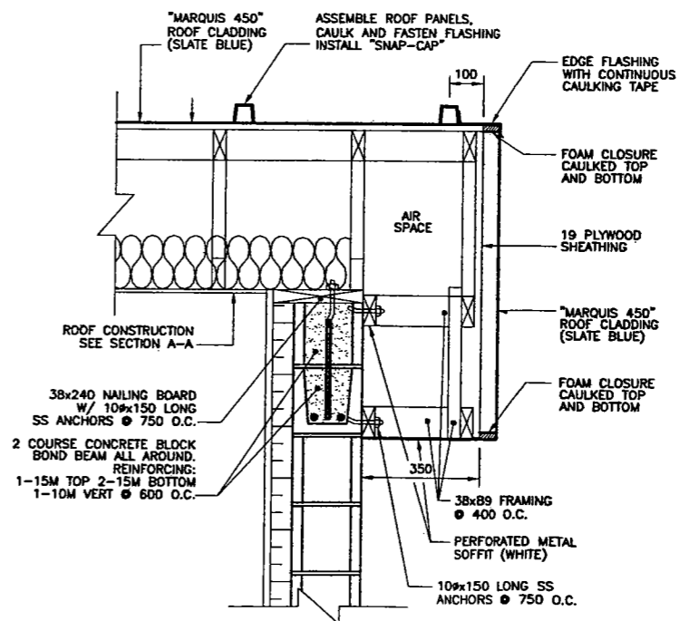
OVERHANG DETAIL SCALE: 1:10
