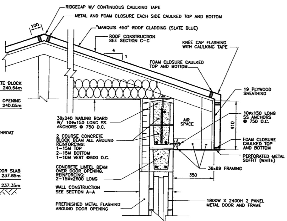
EAVE DETAIL SCALE: 1:10
