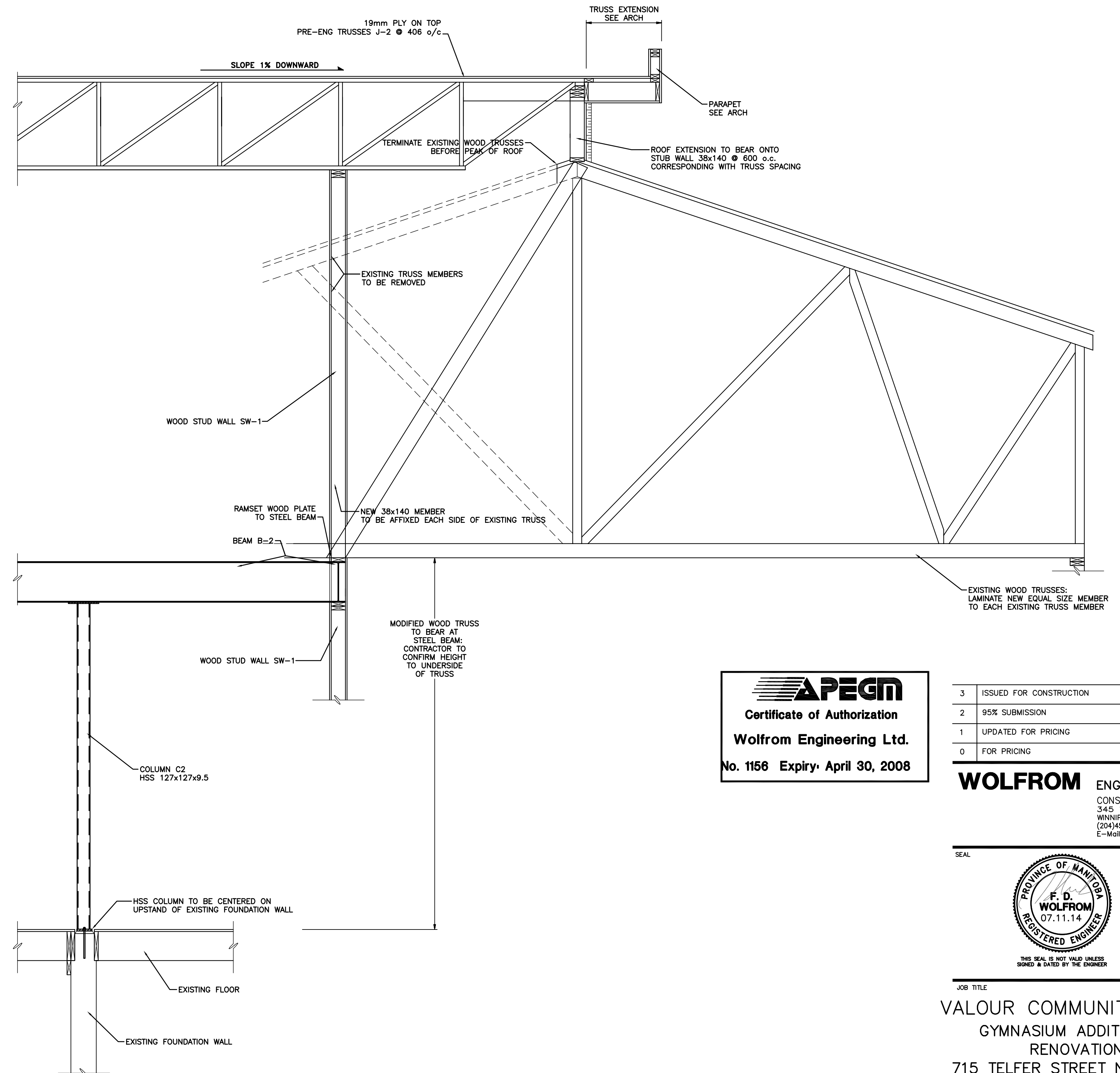
3 SECTION S-5 1 : 25
