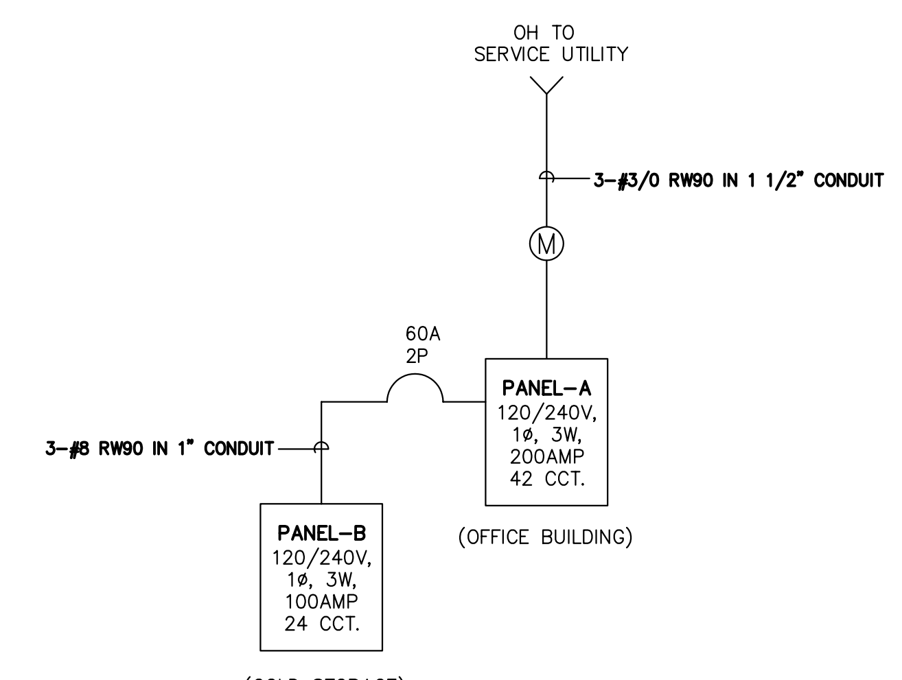
SINGLE LINE DISTRIBUTION SCALE: N.T.S.
