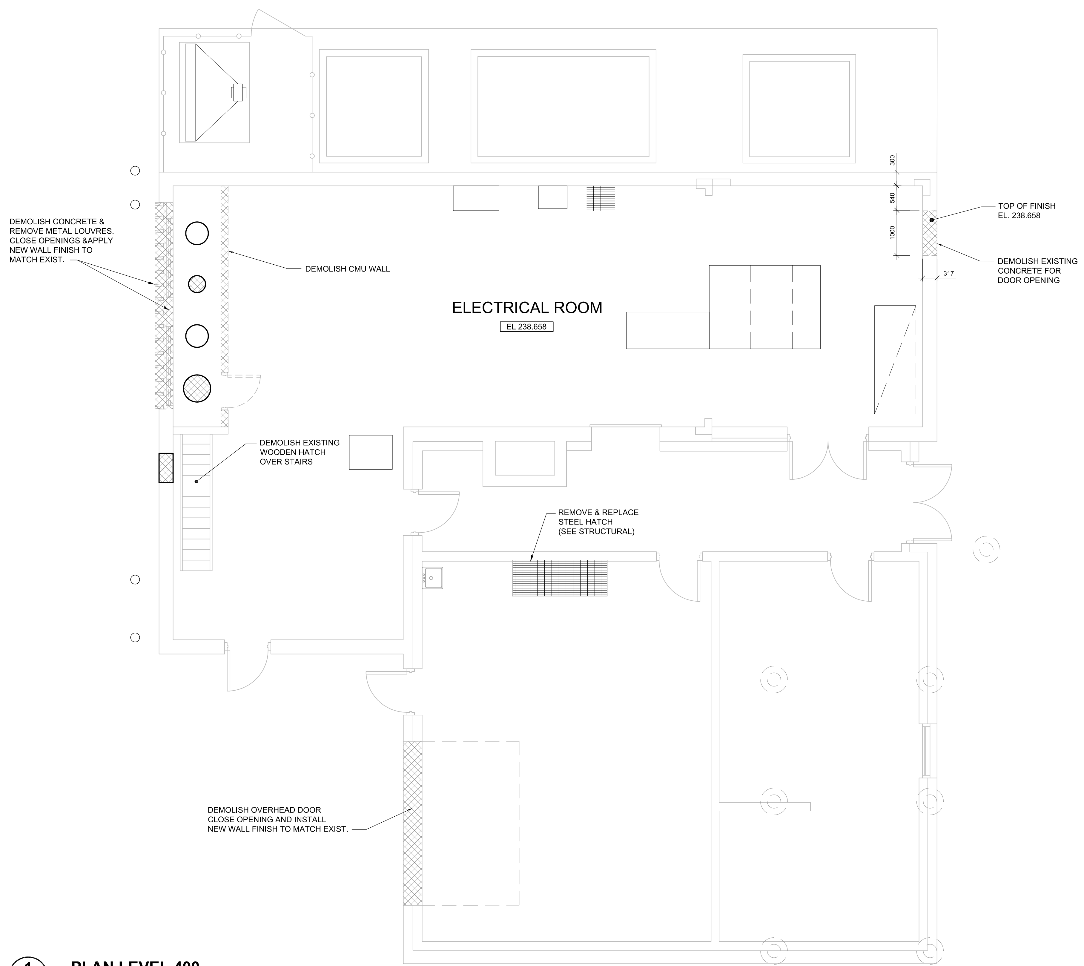
1 PLAN LEVEL 400 A14 SCALE: 1:50
