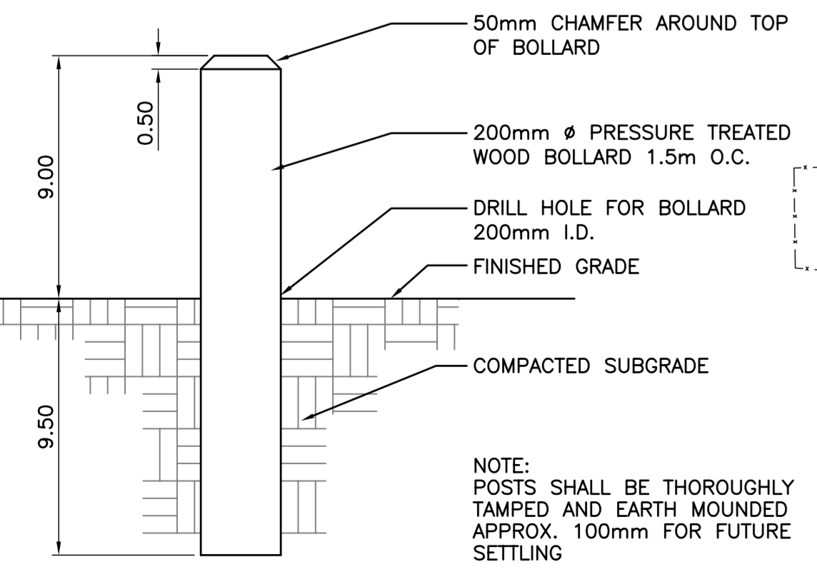
1 WOOD BOLLARD L1 N.T.S.
