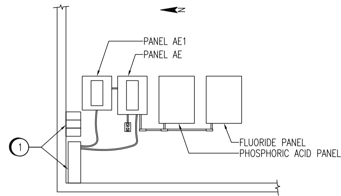
SECTION H SCALE: N.T.S.
