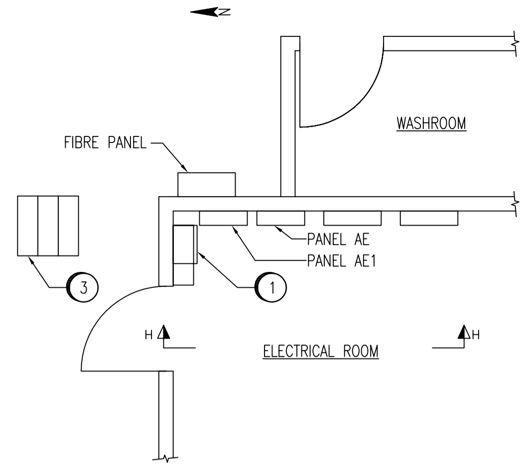
ELECTRICAL ROOM PLAN SCALE: N.T.S.
