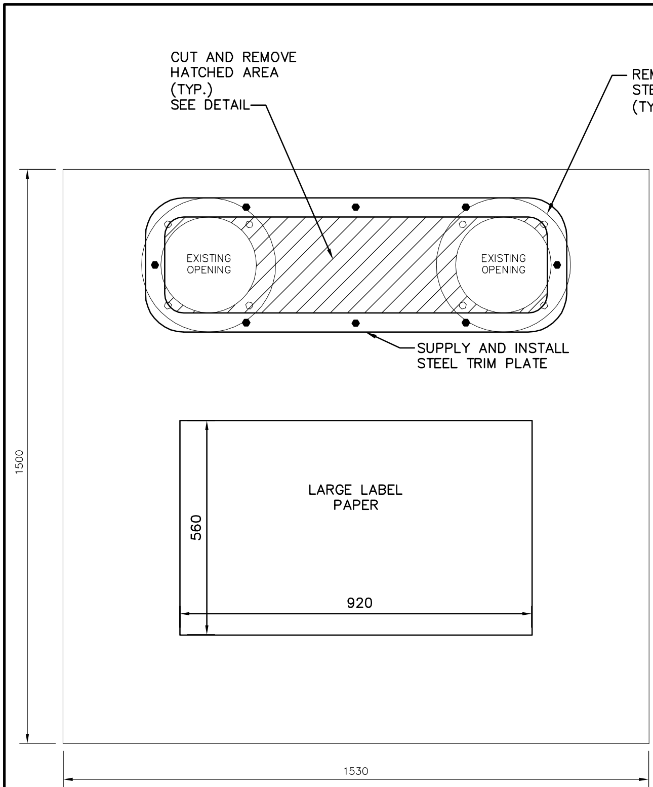
EXISTING CONTAINER AUTOBIN FRONT VIEW N.T.S.
