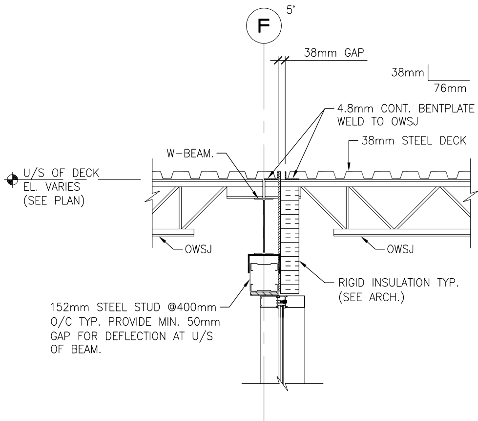
1 SECTION SR-1C SCALE: 1:20
