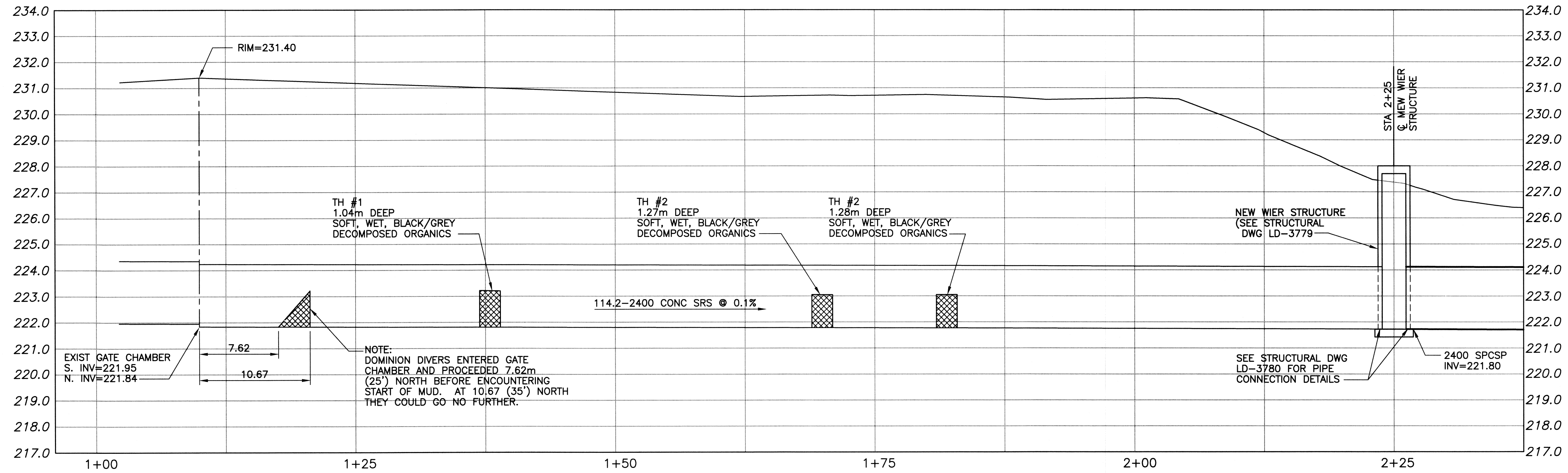
PROFILE SCALE: HOR 1:250 VER 1:100
