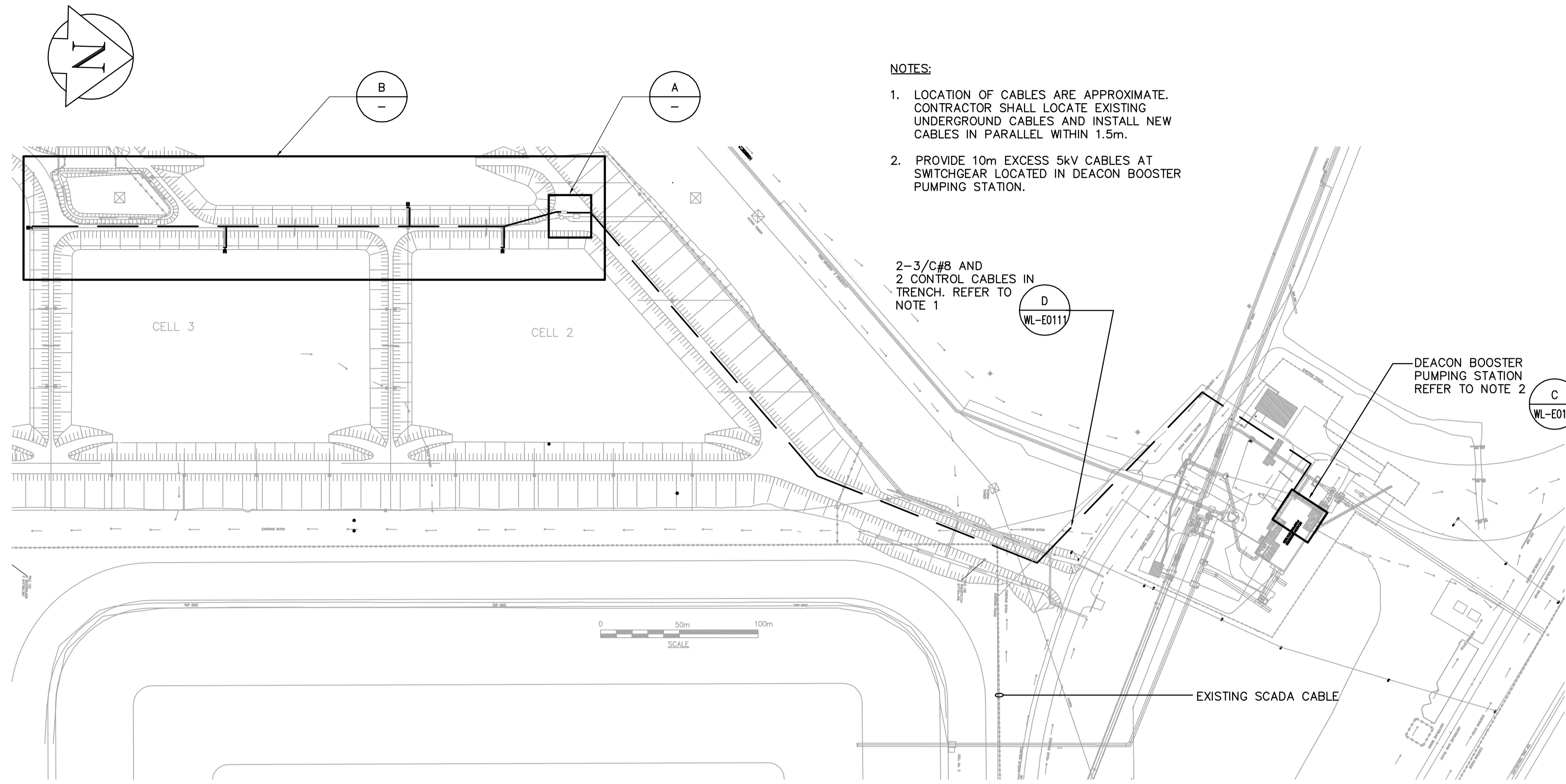
PARTIAL SITE PLAN 1 : 2000
