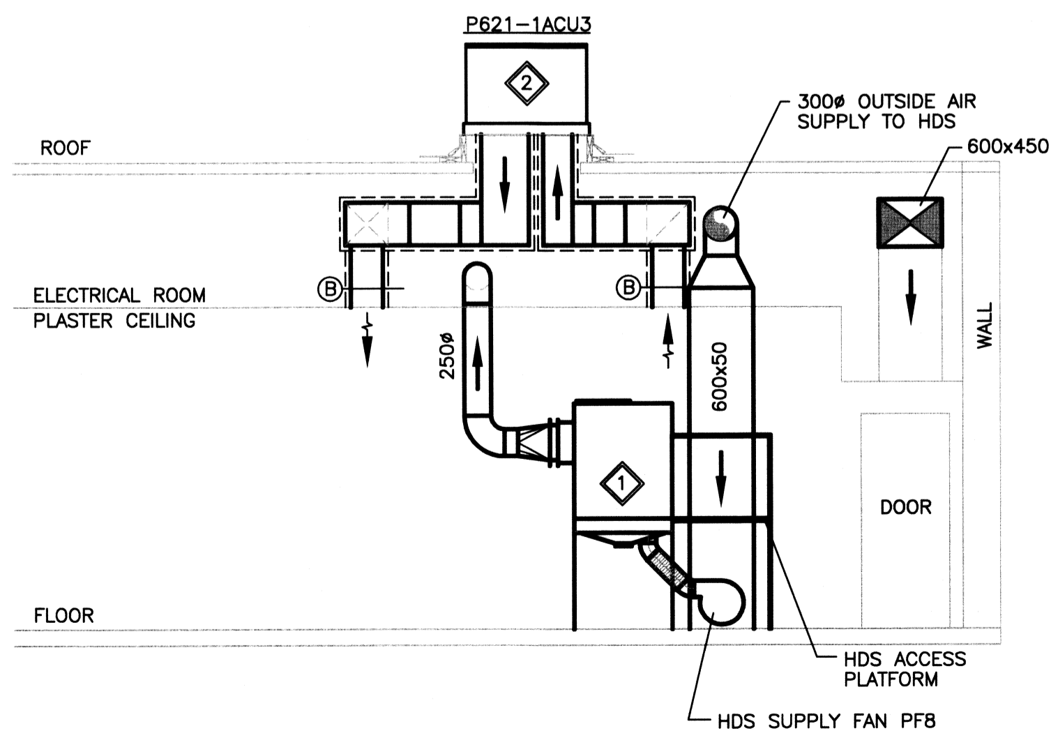
2 SECTION A-A N.T.S.
