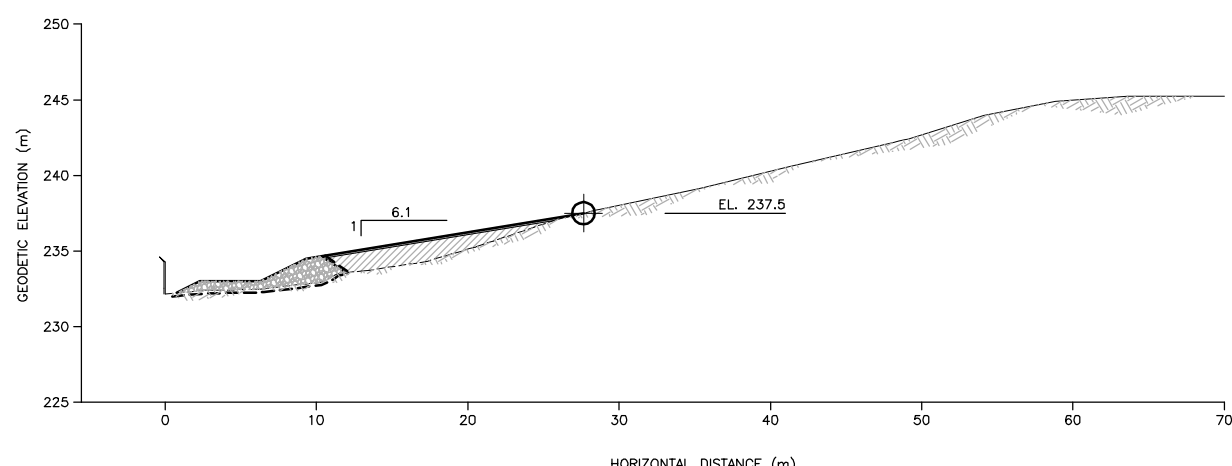
C SECTION (STA 0+248 TO STA 0+285) 01 SCALE: 1:250 (24 x 36") SCALE: 1:500 (11 x 17")
