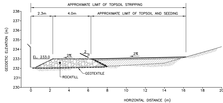
D SECTION 01 SCALE: 1:100 (24 x 36") SCALE: 1:200 (11 x 17")
