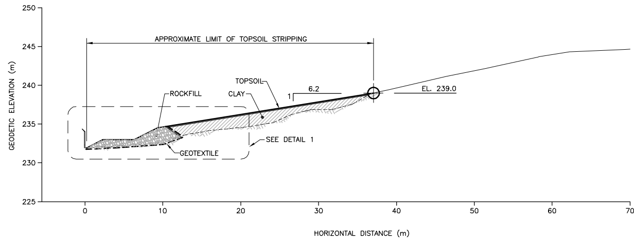
A SECTION (STA 0+090 TO STA 0+138) 01 SCALE: 1:250 (24 x 36") SCALE: 1:500 (11 x 17")
