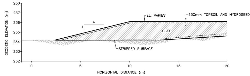
E SECTION 01 SCALE: 1:100 (24 x 36") SCALE: 1:200 (11 x 17")
