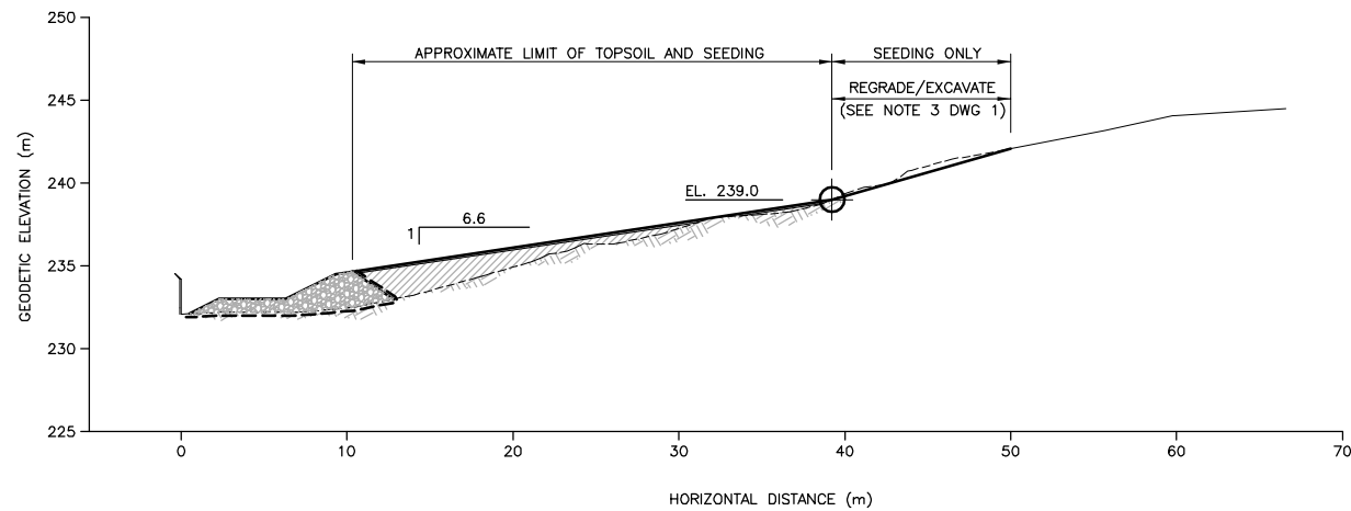
B SECTION (STA 0+175 TO STA 0+230) 01 SCALE: 1:250 (24 x 36") SCALE: 1:500 (11 x 17")
