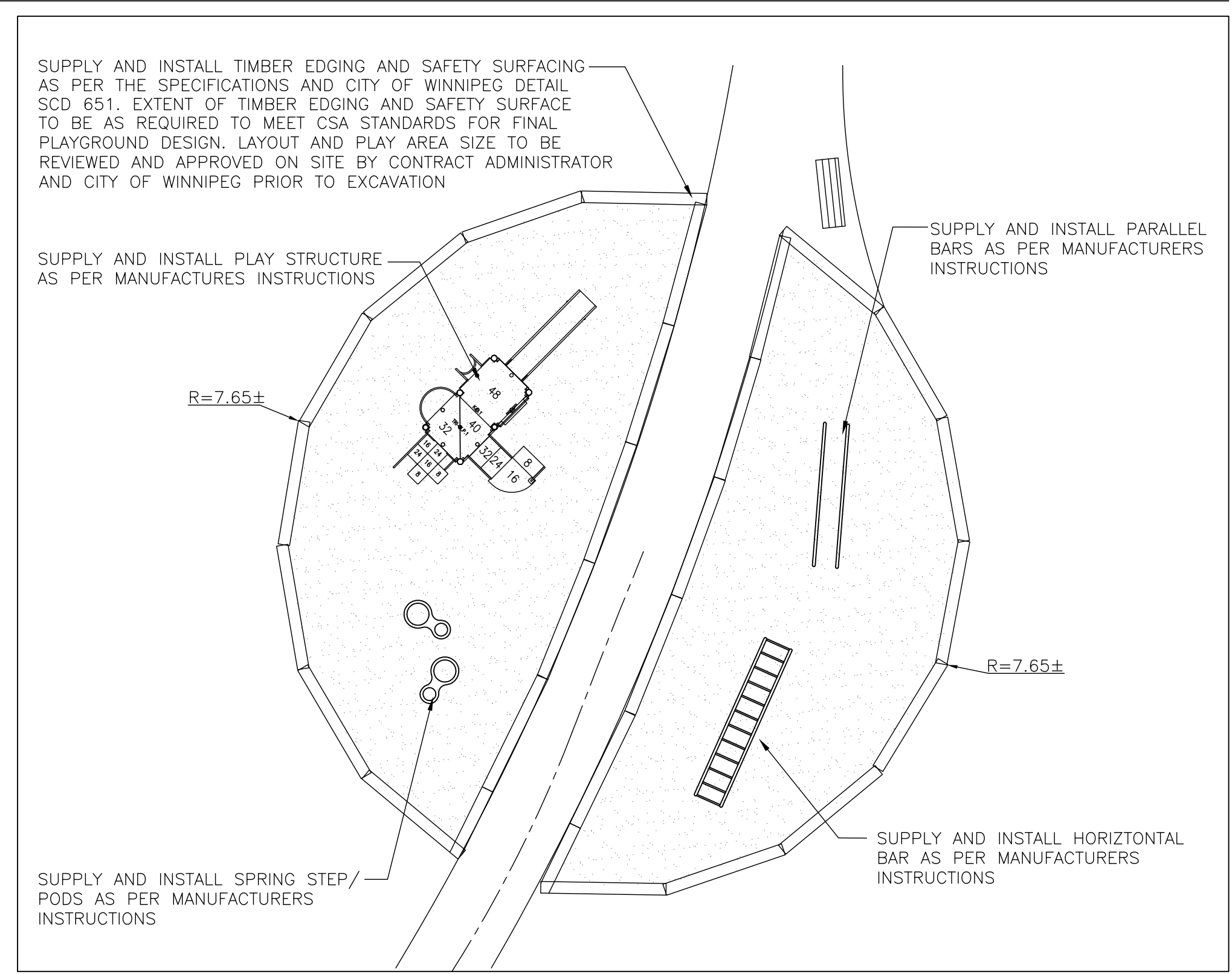
ENLARGEMENT 1 SCALE 1:100
