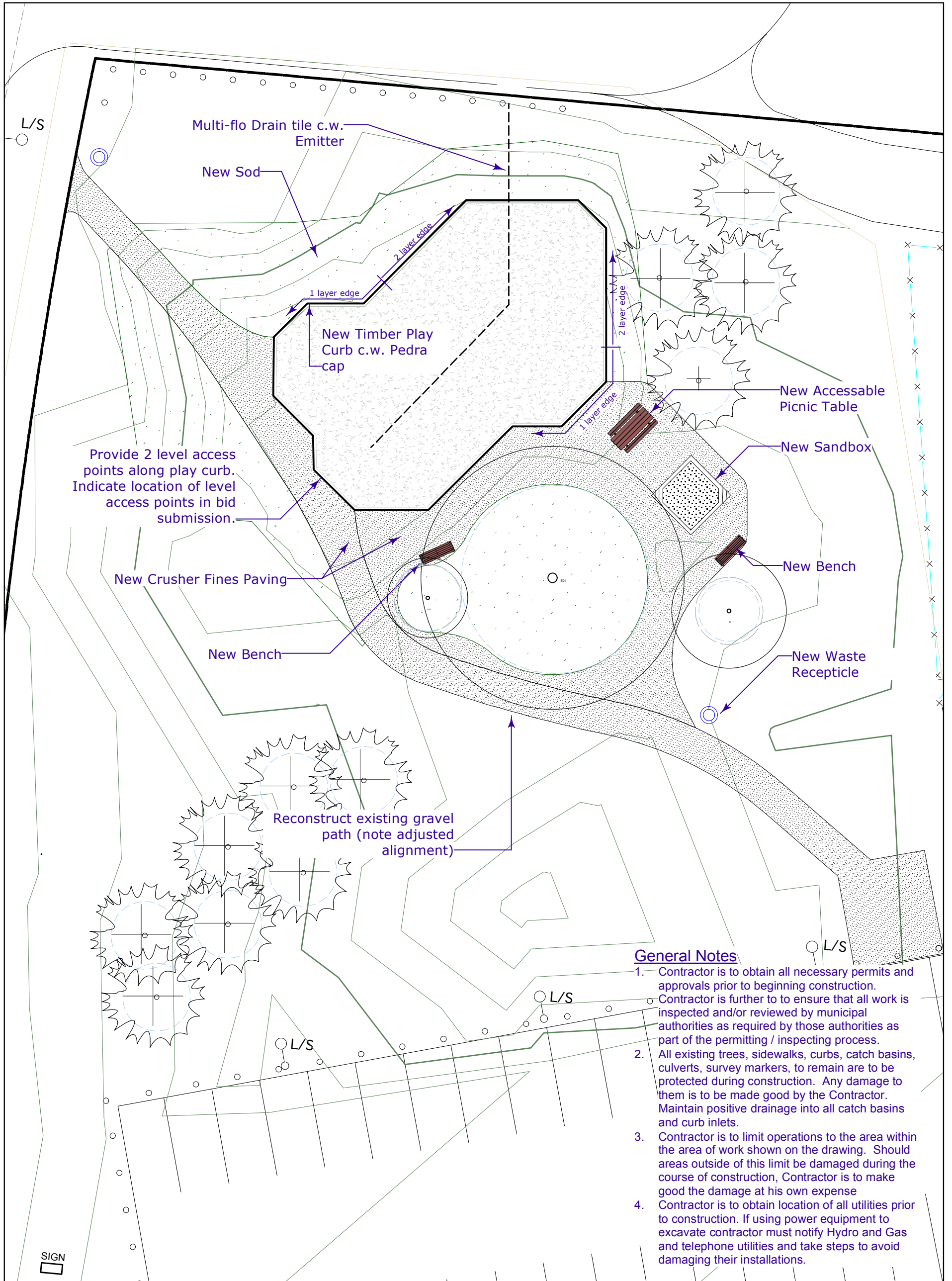
1 Layout Plan L-5 Scale: 1:200
