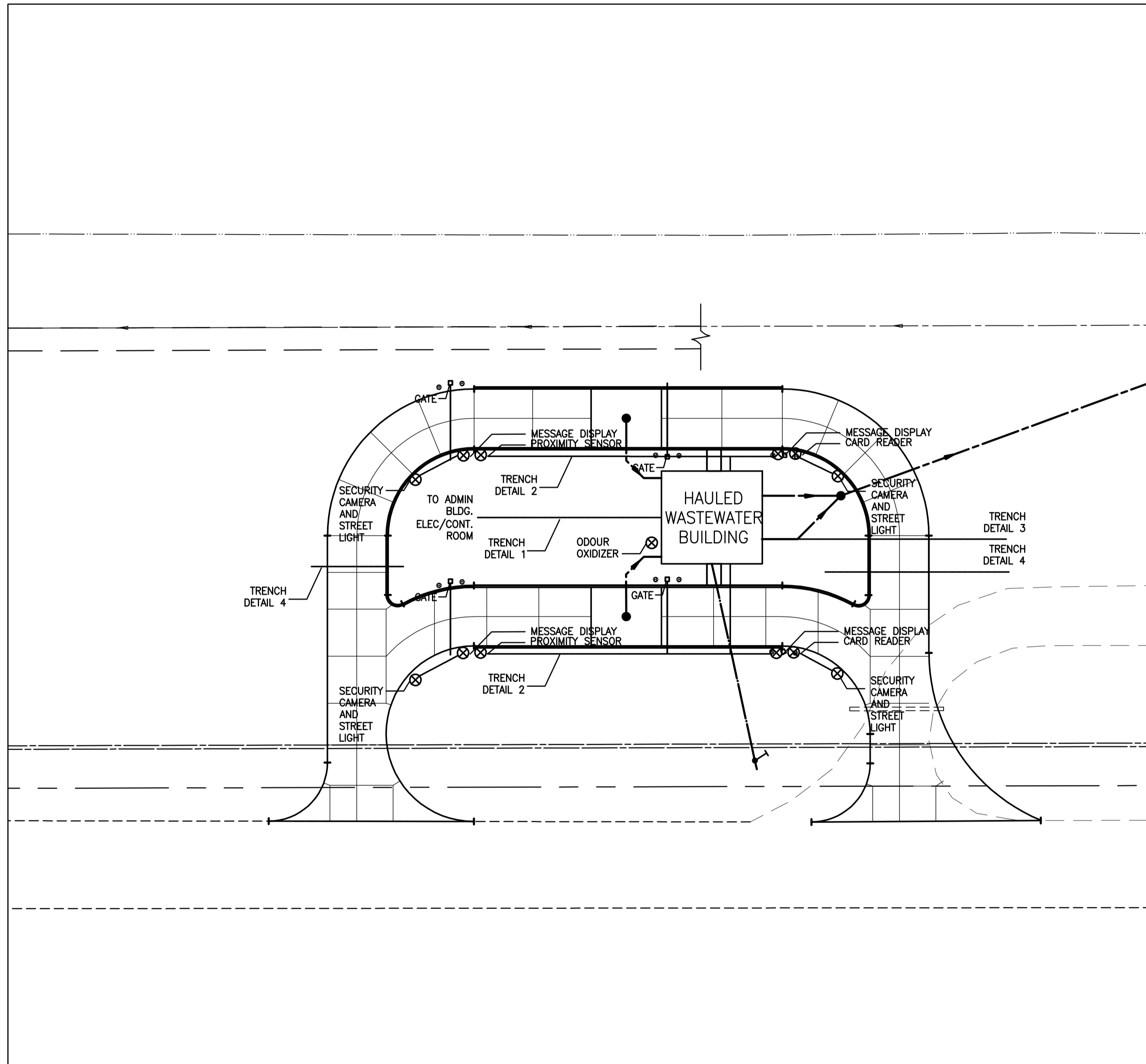
SITE PLAN 1:250
