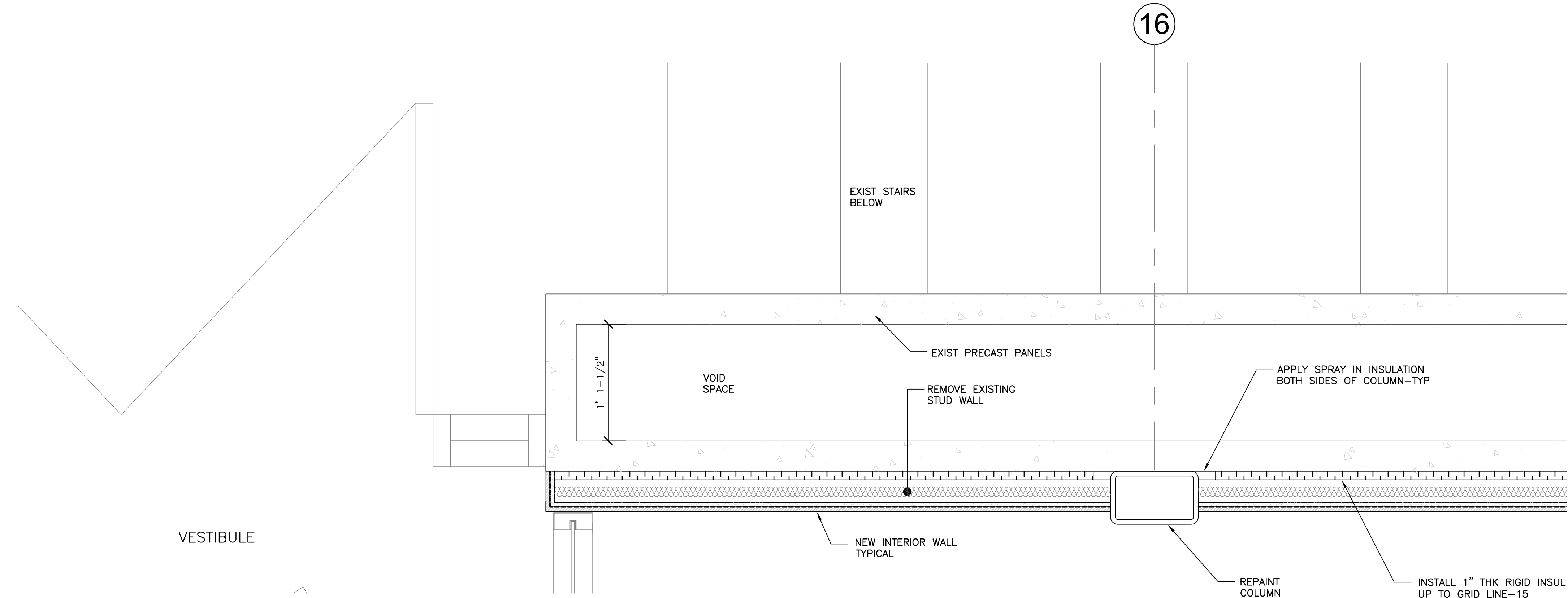
2 SE VESTIBULE WALL DETAIL SCALE: 1 1/2"=1'-0"
