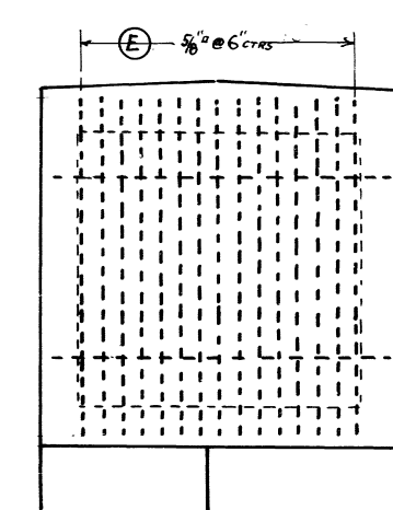
END ELEVATION
