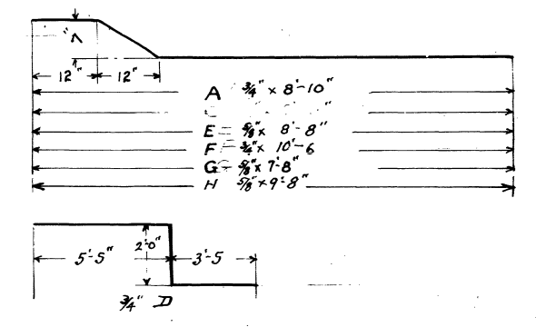
SECTION D-D
