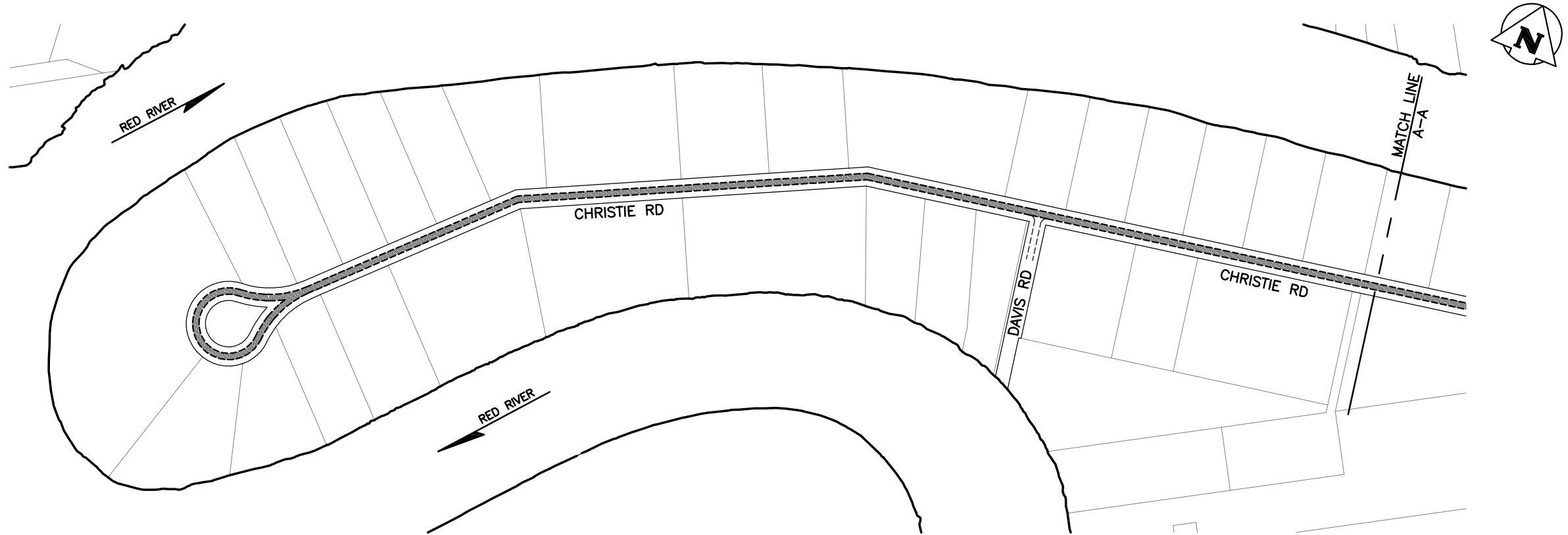
PLAN - CHRISTIE RD SCALE: 1:2500
