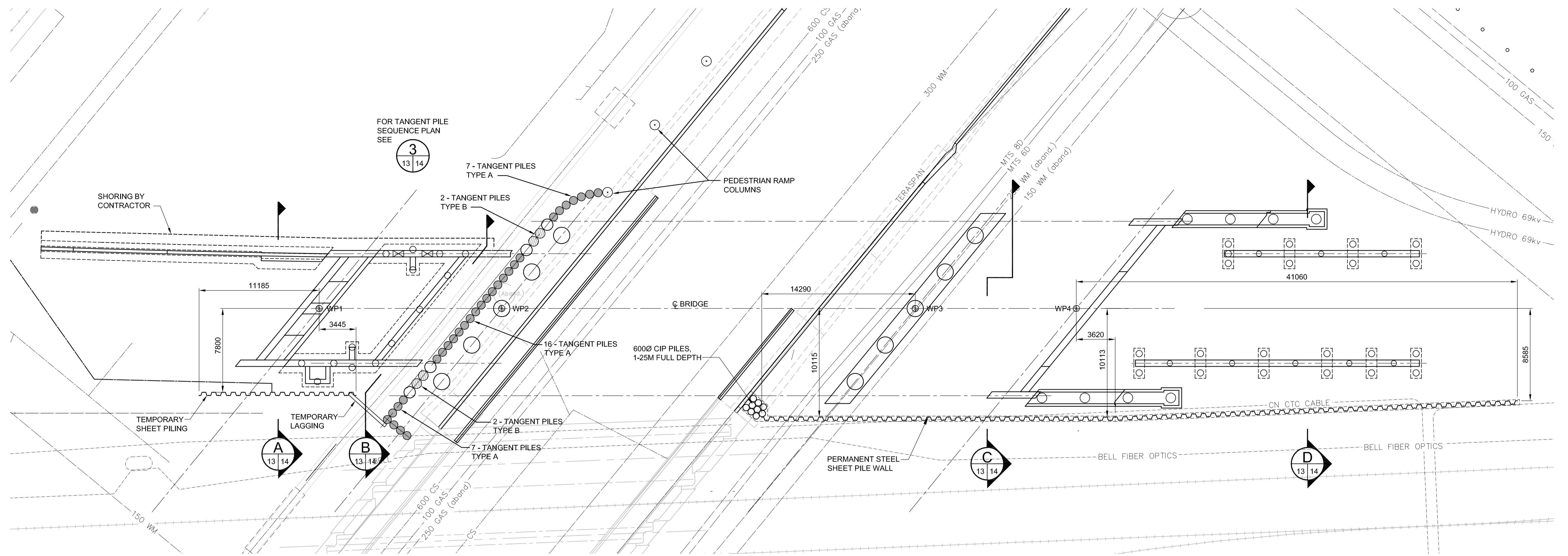
PLAN SCALE: 1:200
