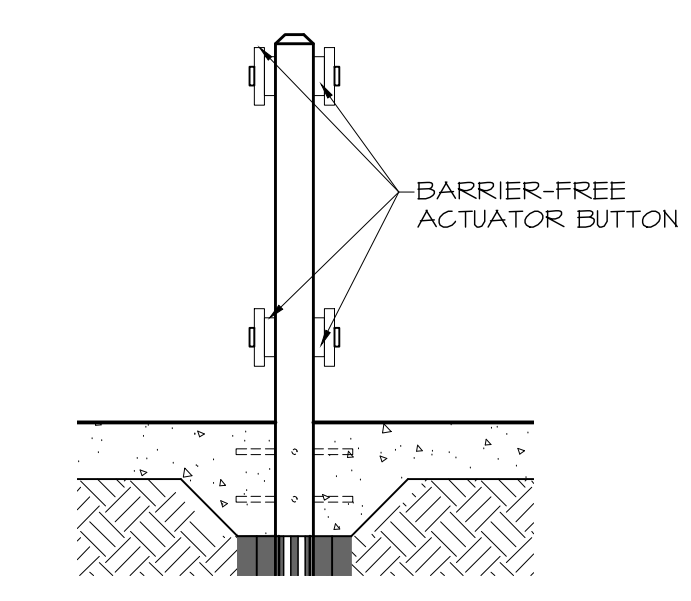
4 B.F. DOOR ACTUATOR SIDE ELEV 2.1 | 2.1 1:20
